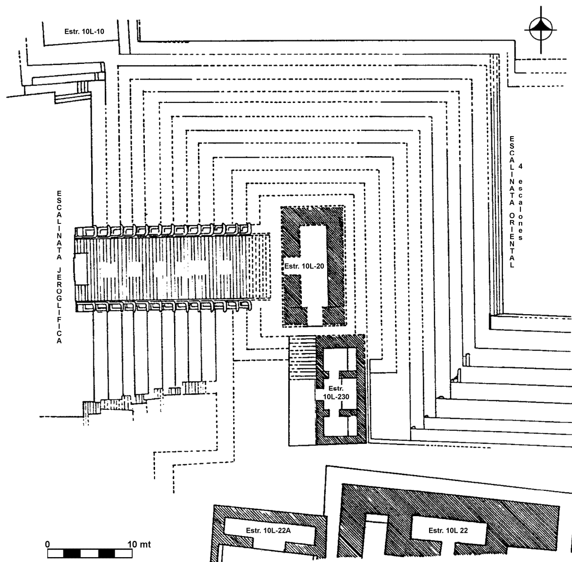
Figura 3 Planta de la estructura 10L-26, por Rudy Larios V.
