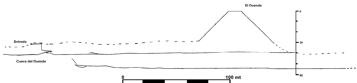
Figura 3 Sección de la Cueva de Río El Duende y de la Cueva de El Duende
