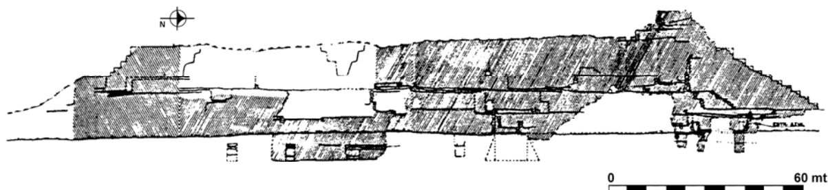
Figura 4 Copan, Acrópolis, alzado esquemático mostrando áreas consolidadas
