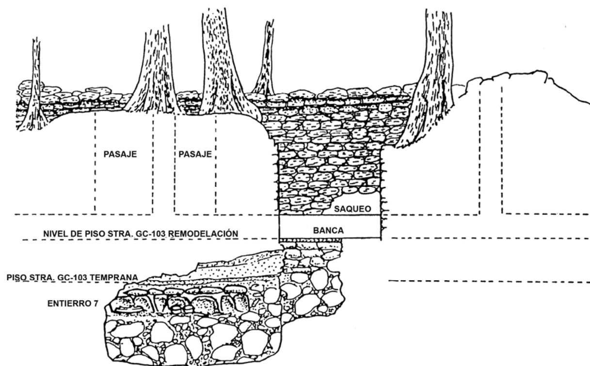
Figura 5 Elevación este mostrando el detalle del Entierro 7
