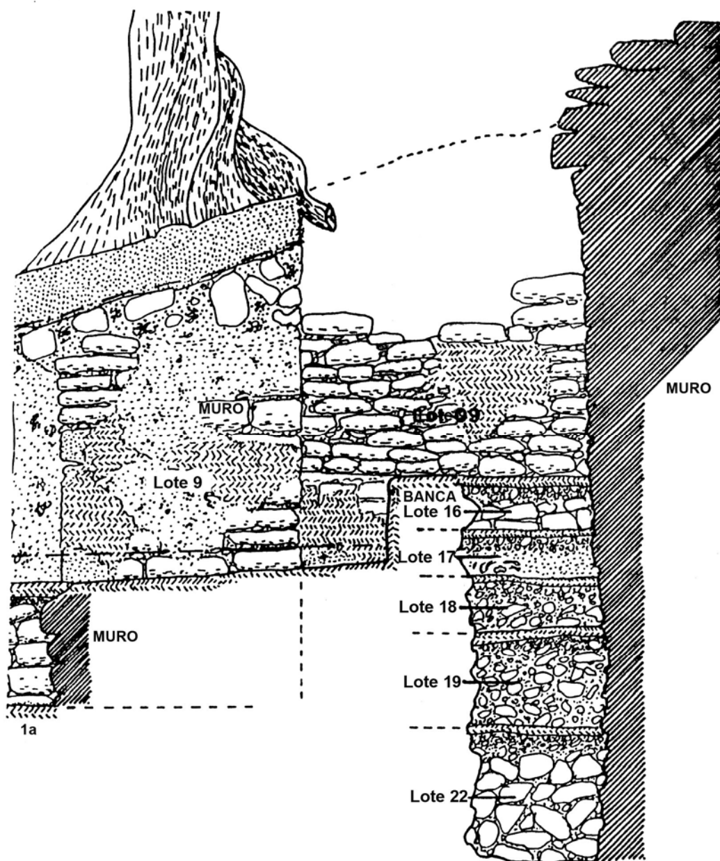
Figura 3 Perfil norte mostrando los gruesos muros interiores de las cámaras
