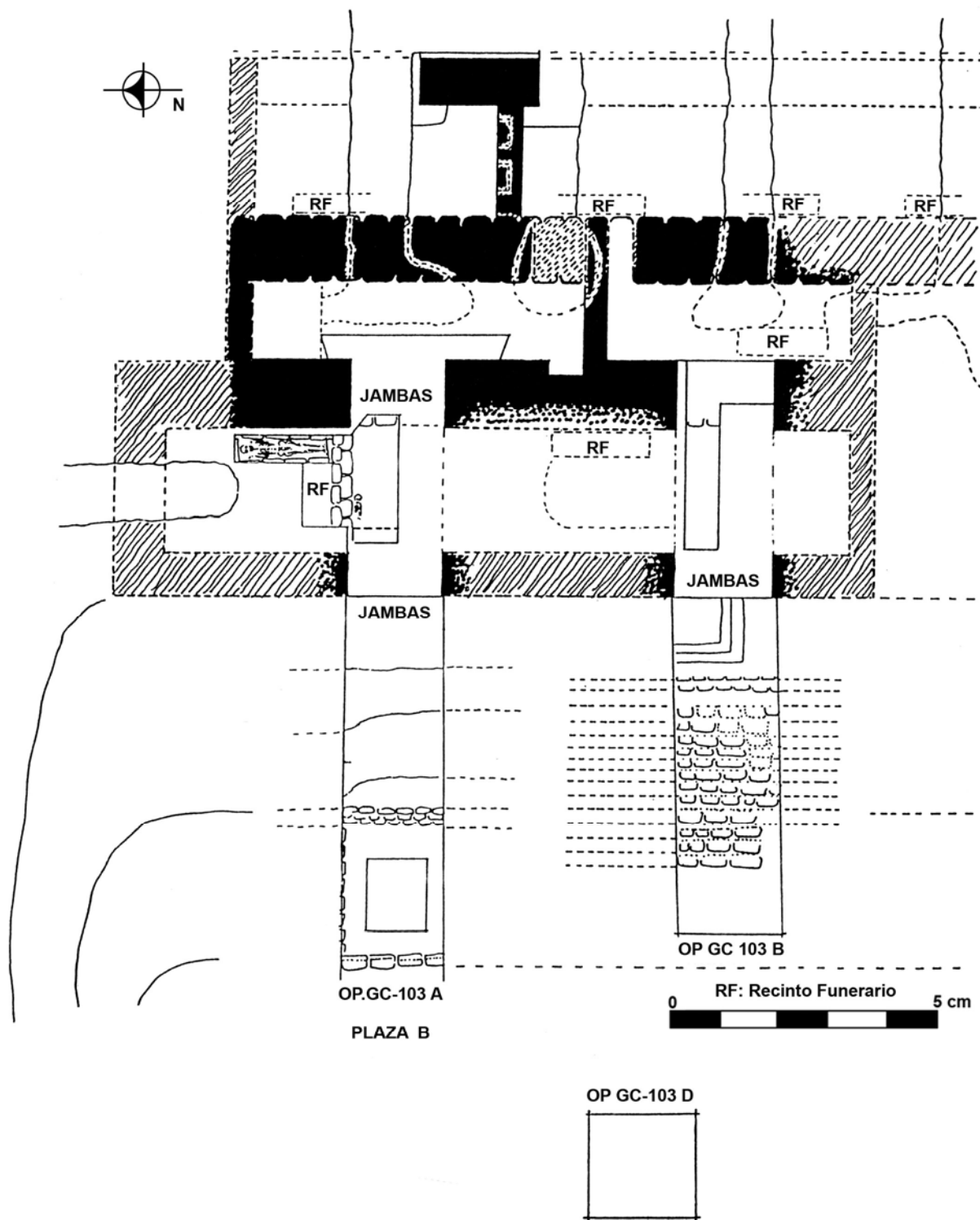
Figura 4 Planta general indicando las jambas y accesos a las cámaras interiores. Nótese la ubicación de recintos funerarios
