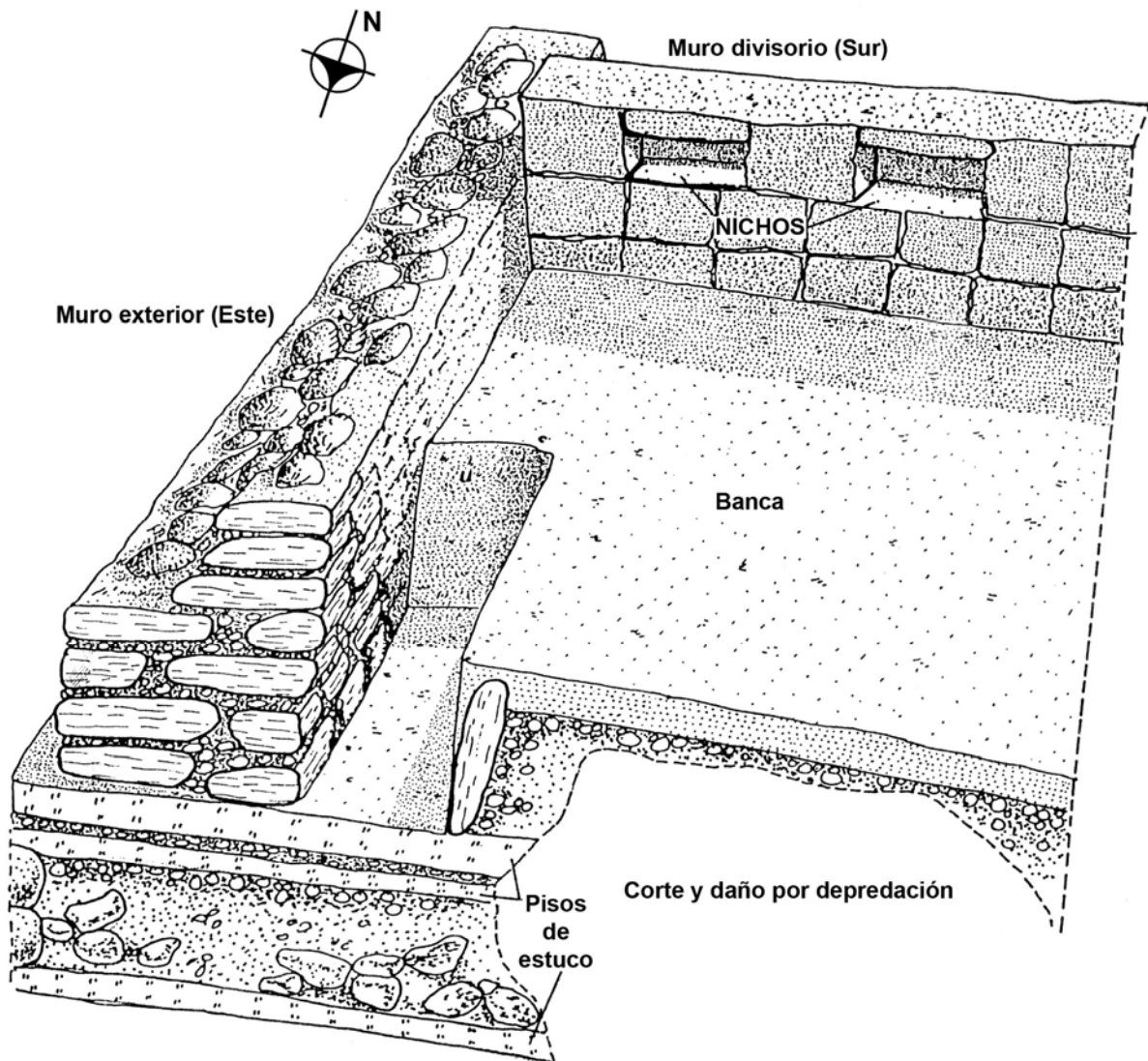
Figura 14 Isométrica del área restaurada mostrando el trabajo realizado en los muros, nichos y bancas restaurados
