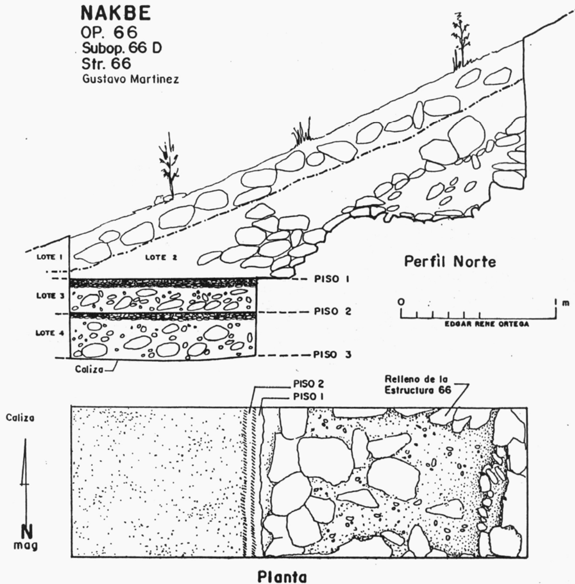
Figura 12 Perfil este de la Operación 66 D, indicando los pisos sucesivos del callejón entre las Estructuras 59 y 66
