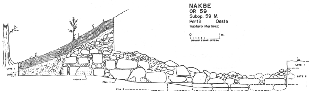
Figura 11 Perfil norte de la Operación 59 M, revelando la esquina y la fachada oriental de la Estructura 59. Se notan las piedras grandes puestas por la base de la estructura
