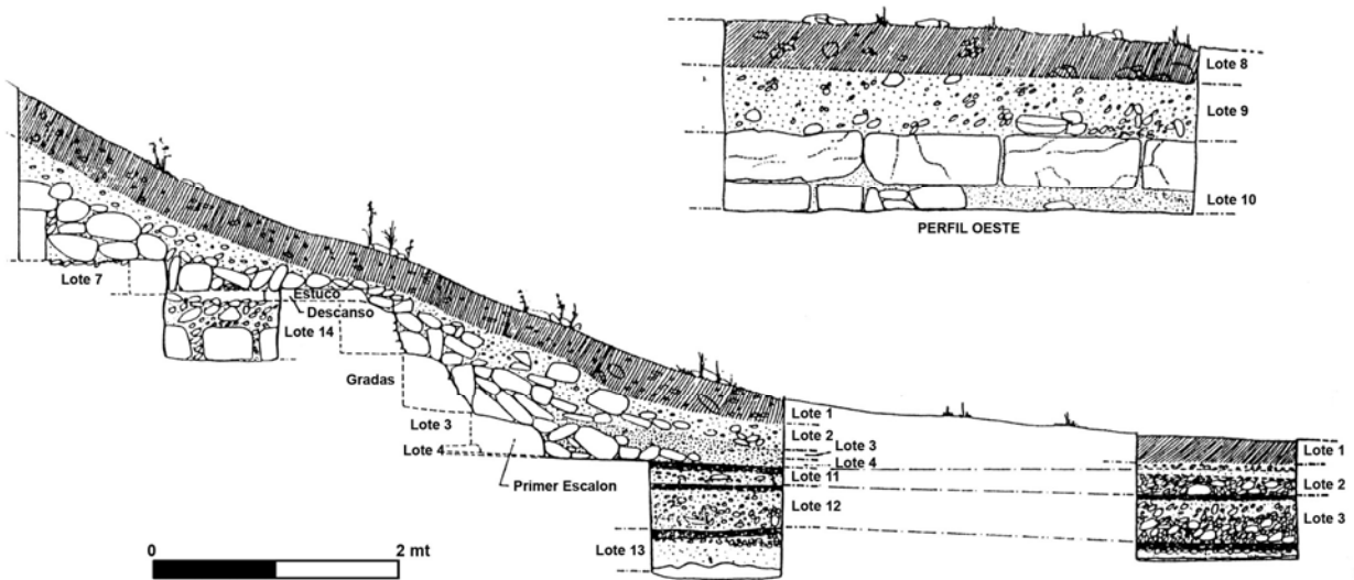
Figura 8 Perfil sur de la Operación 59 K al investigar el callejón entre las Estructuras 59 y 51. Se notan los tres pisos sucesivos
