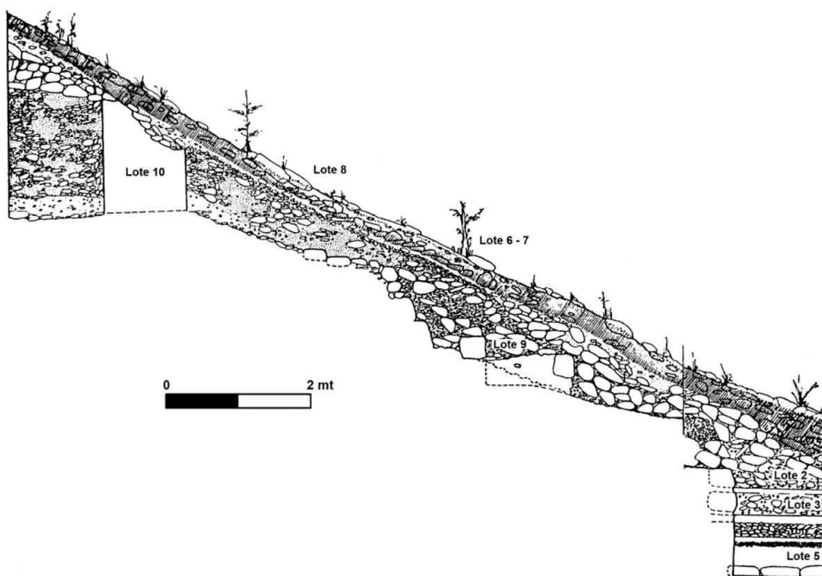
Figura 4 Perfil sur de la Operación 59 K. Se notan los cuatro pisos de la construcción
