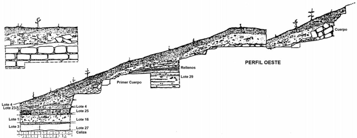
Figura 9 Perfil norte de la excavación inferior de la Operación 59 H, ubicado por la fachada sur de la Estructura 59. Se notan los pisos por el callejón entre las Estructuras 59 y 66
