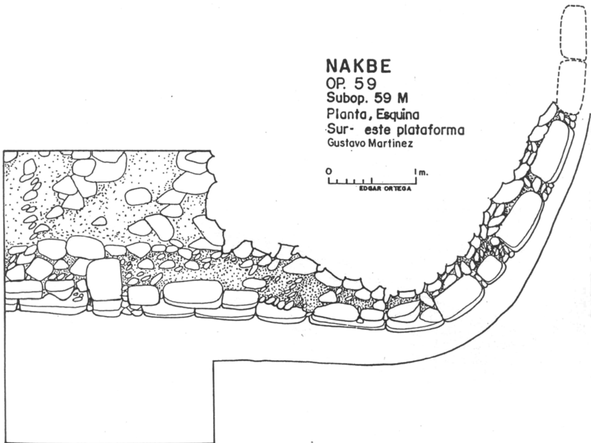
Figura 10 Esquina sureste de la Estructura 59, la Operación 59 M, indicando la forma redondeada
