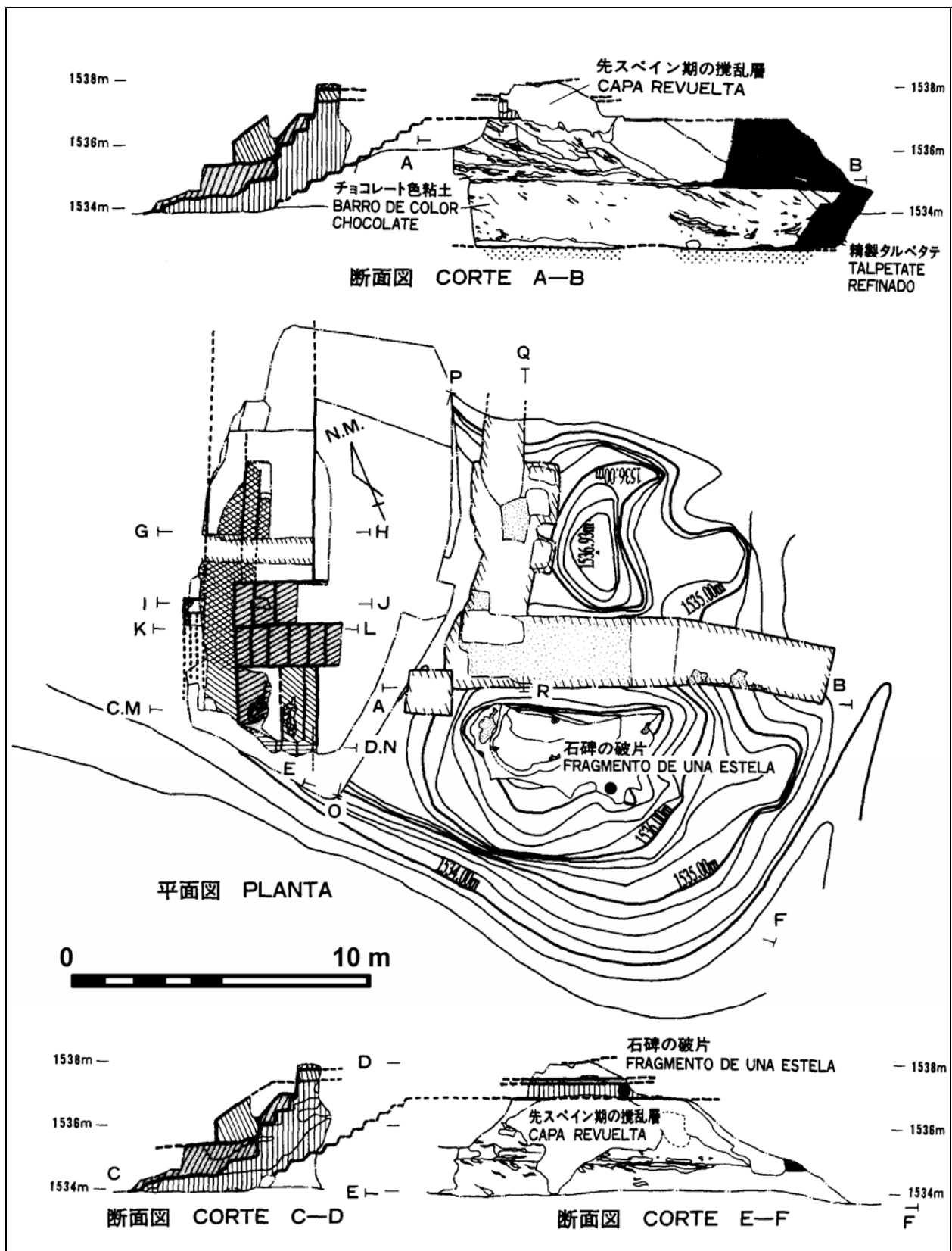
Figura 4 Corte de la Estructura D-III-1
