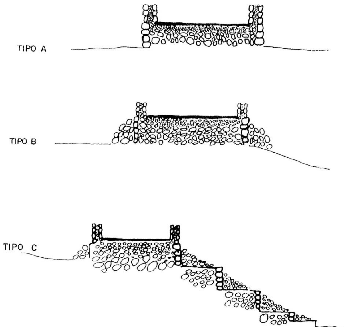
Figura 2 Tipos constructivos de calzadas: A) Tipo A; B) Tipo B; C) Tipo C
