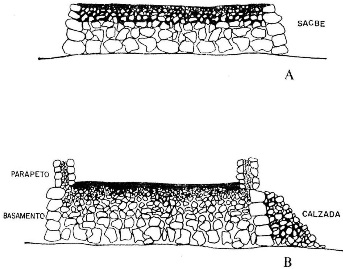
Figura 1 A) Perfil de un sacbe; B) Perfil de una calzada señalando el basamento y los parapetos
