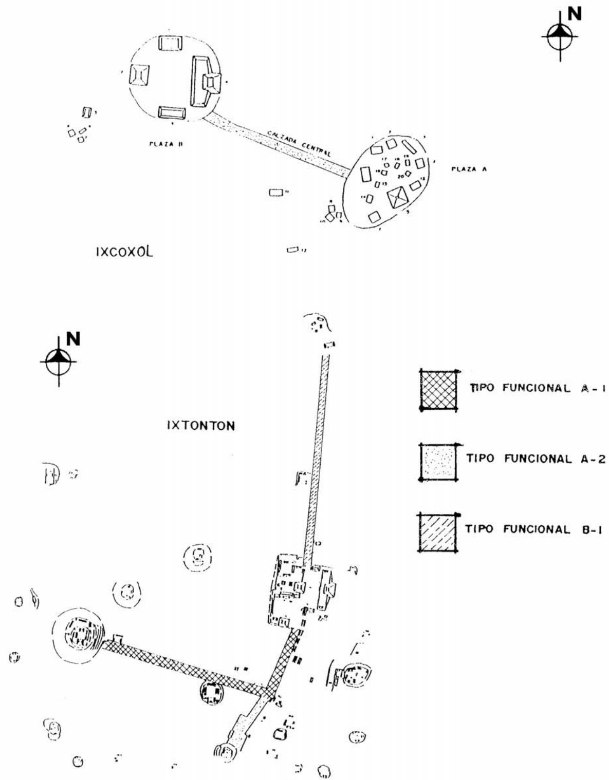
Figura 3 Calzadas de Tipo Funcional de Cohesión Urbanística A-1 y A-2, Mapas de Ixtonton e Ixcxol
