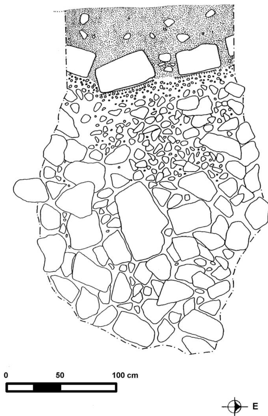
Figura 5 Perfil de excavación de saqueo, lado norte, Estructura 7, Punta de Chimino
