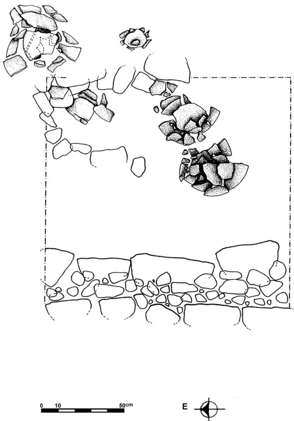
Figura 9 Planta de excavación, Escondite 1, Estructura 7, Punta de Chimino
