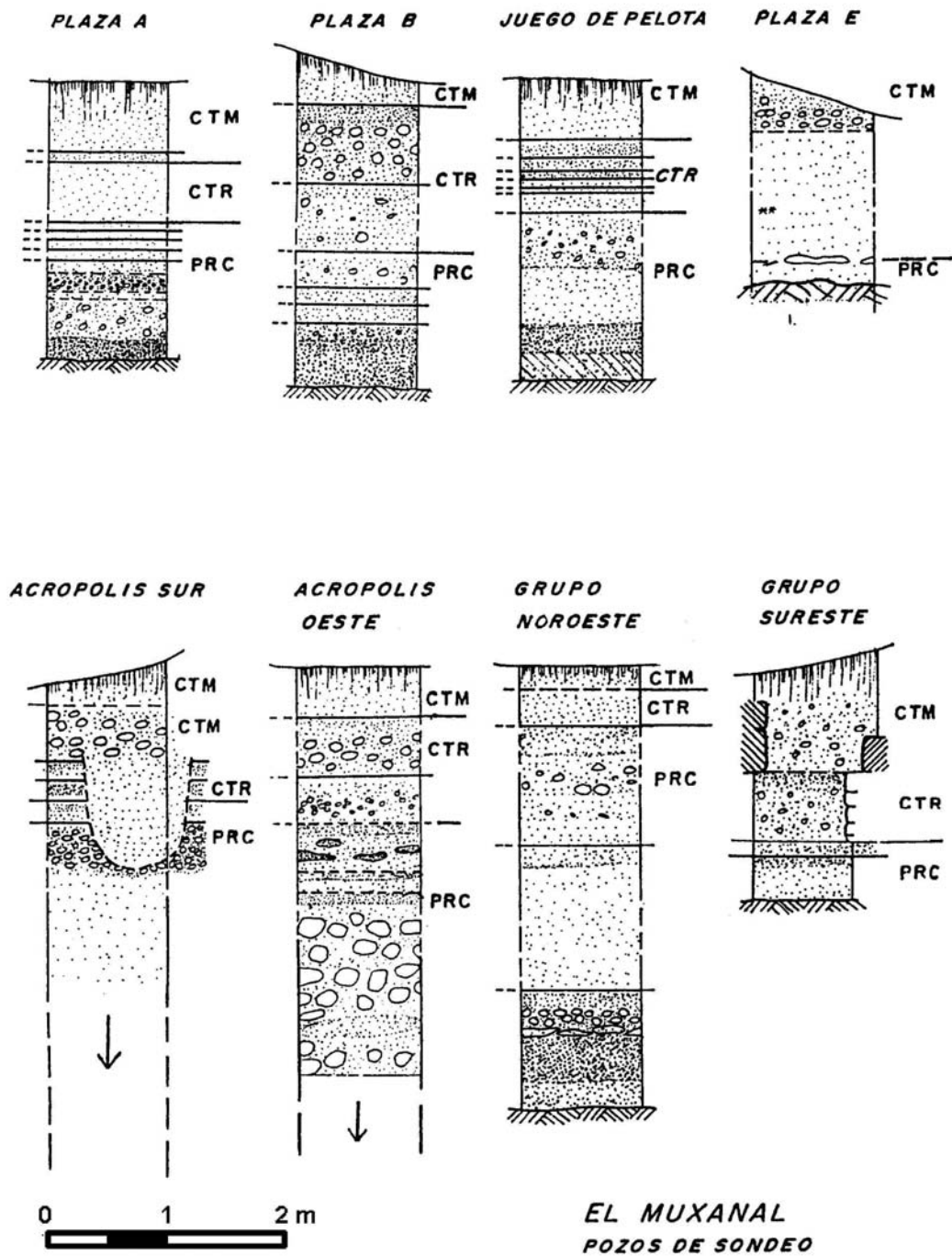
Figura 5: Estratigrafía de los pozos de sondeo (Dibujo: Paulino Morales)
