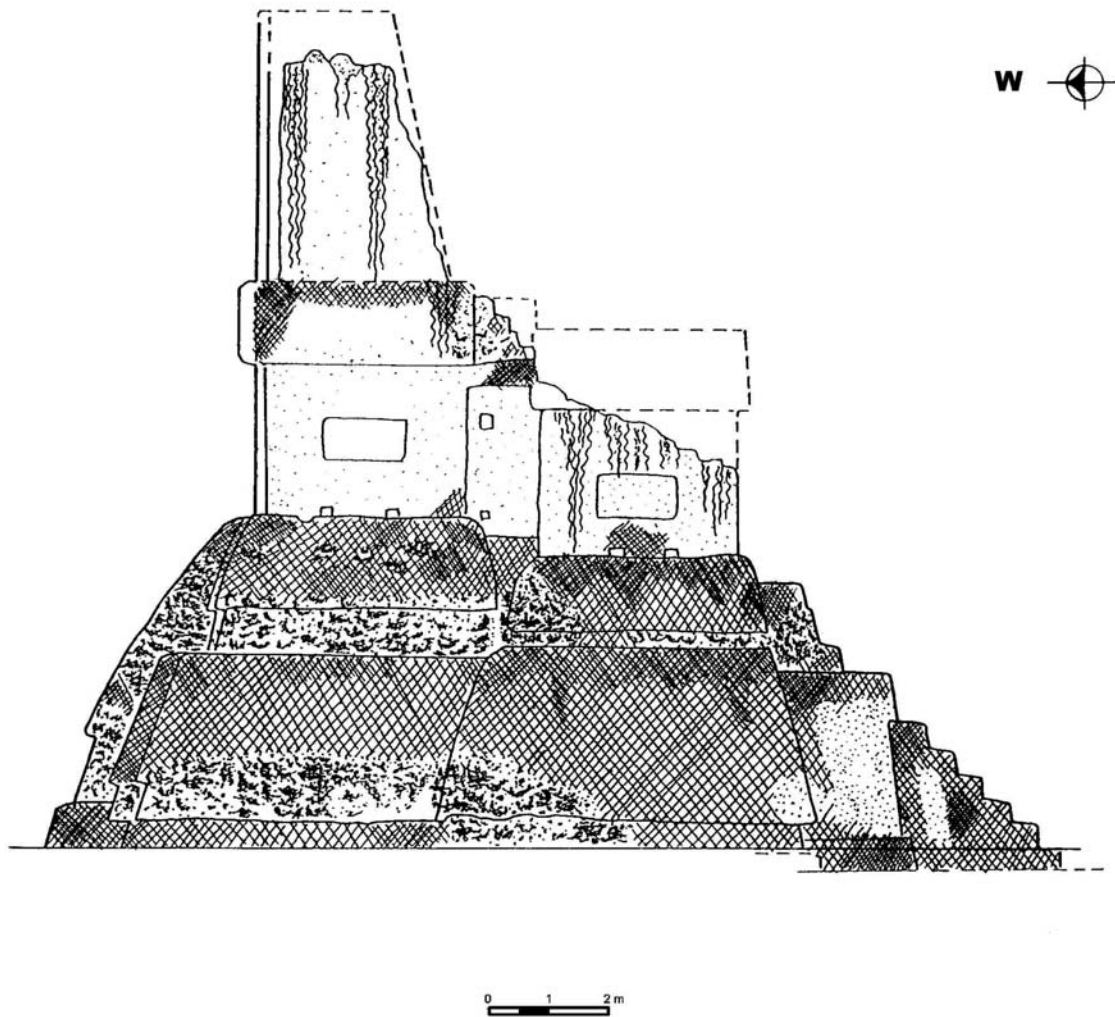
Figura 3 Proyecto de Conservación Tikal - Etapa I, 1996: Estructura 5D-23-2, Fachada Sur, Escala 1:100, dibujo Ivo Romero
