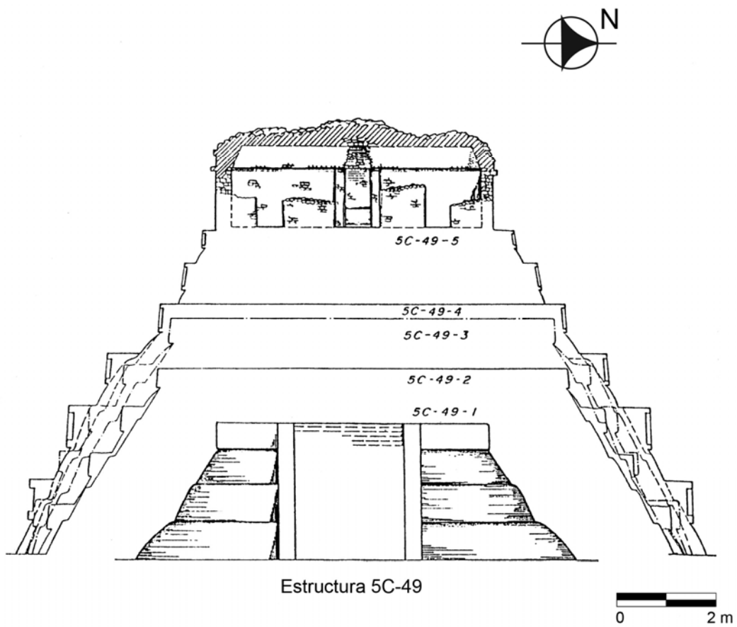
Figura 4 Corte norte-sur de 5C-49
