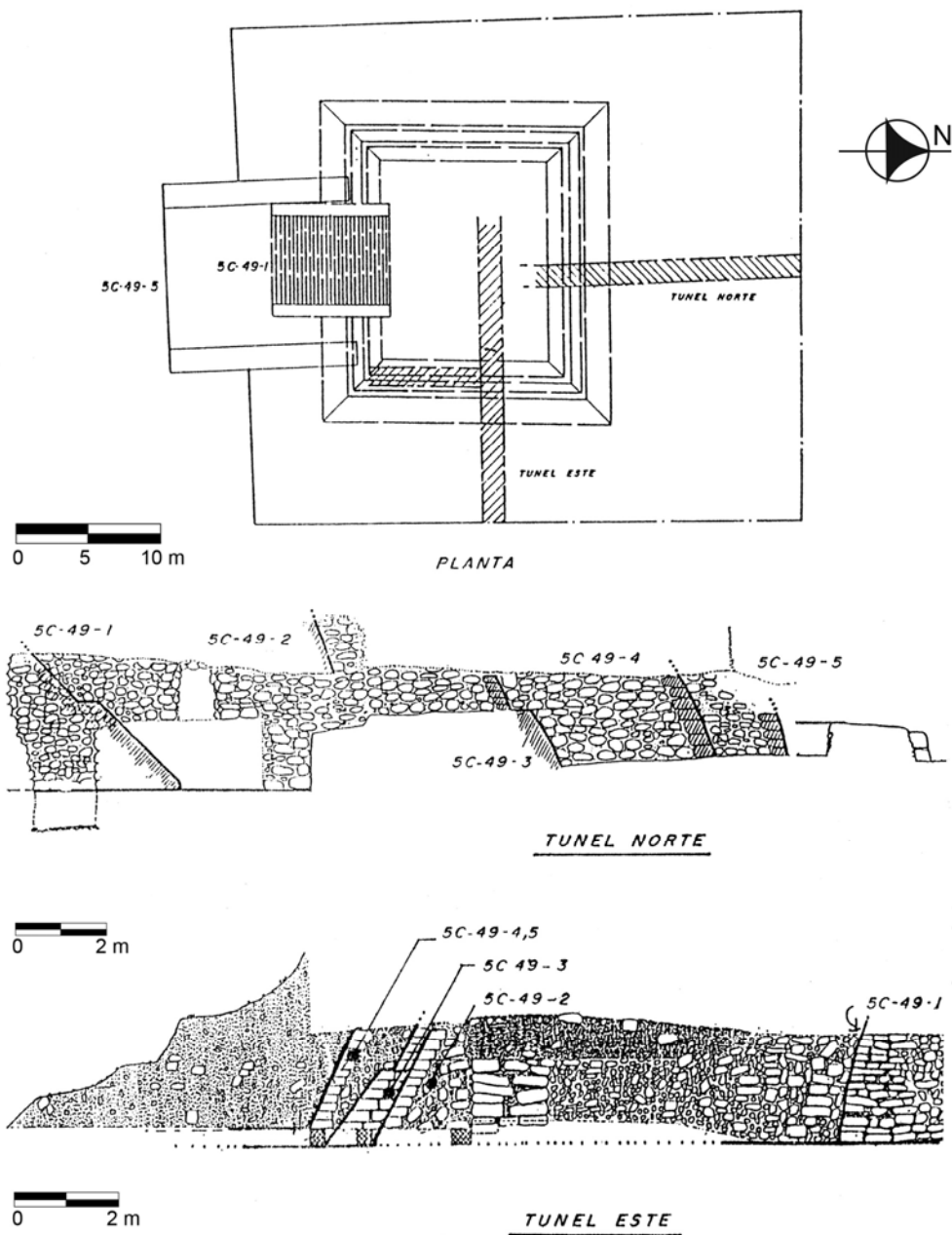
Figura 3 Planta y perfiles de los túneles perforados dentro de 5C-49
