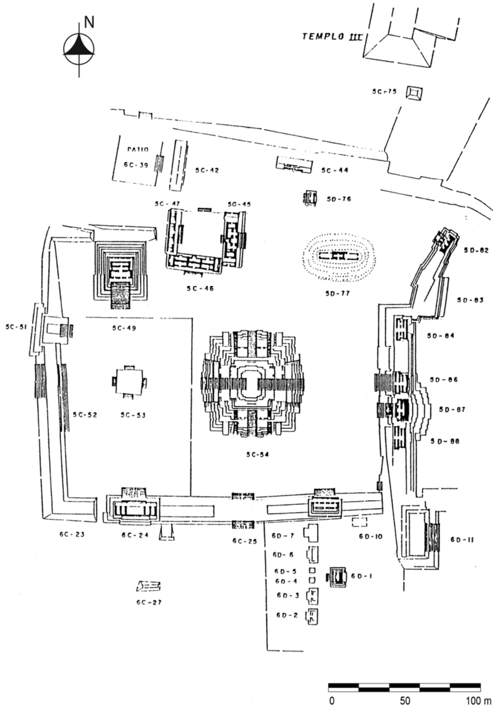
Figura 2 Plano de Mundo Perdido en el Clásico Tardío
