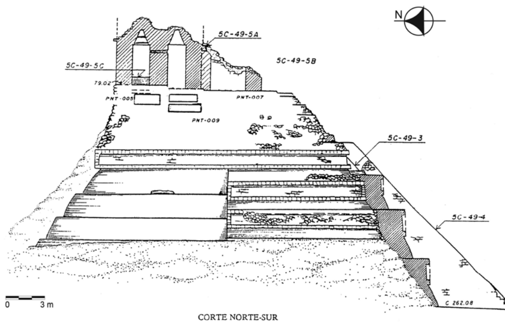
Figura 8 Corte norte-sur, lado oeste, de 5C-49
