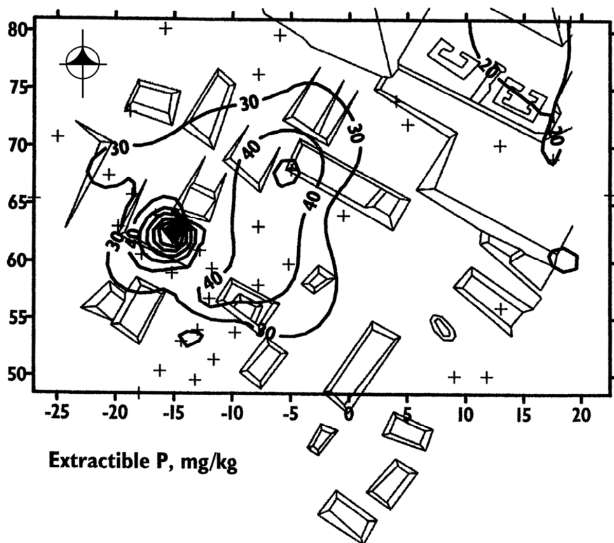
Figura 1 Ubicación de muestras de suelos de los Grupos O y N, residencial sub-élite y los contornos de concentración P extraíble Mehlich II
