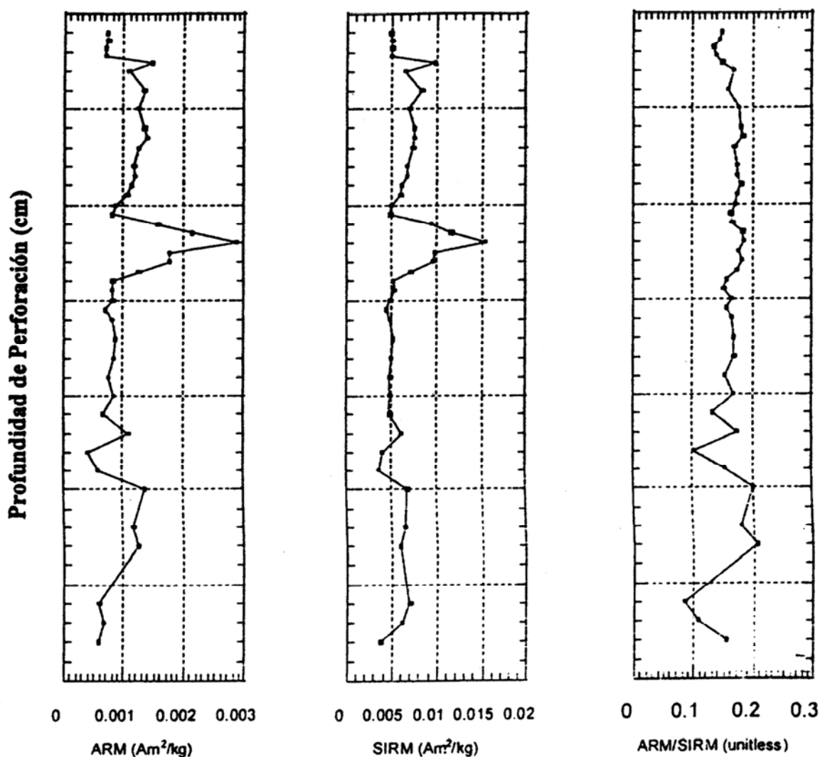
Figura 3 Los análisis ARM y SIRM de la muestra de la laguna Las Pozas
