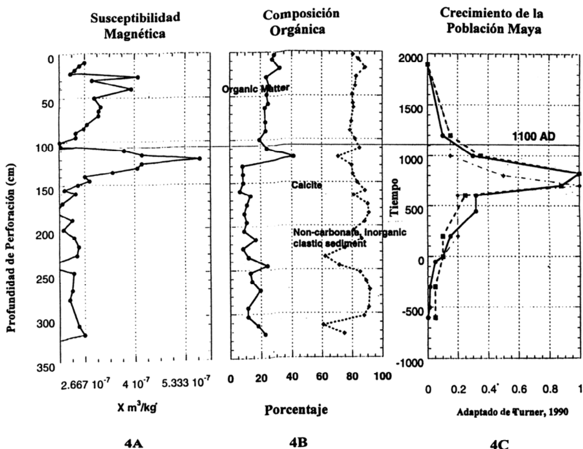
Figura 4 Índices de la muestra de la laguna Las Pozas: 4a Susceptibilidad magnética; 4b Composición orgánica; 4c Comparación del crecimiento de la población Maya del periodo Clásico Tardío (adaptado de Turner 1990) y el índice de la susceptibilidad magnética
