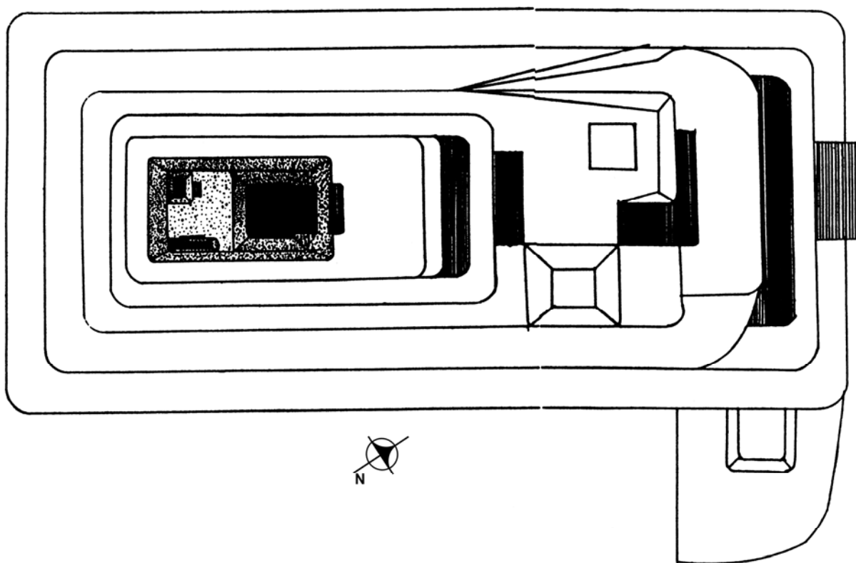
Figura 11 Planta general de la pirámide principal de Chaak Ak'al
