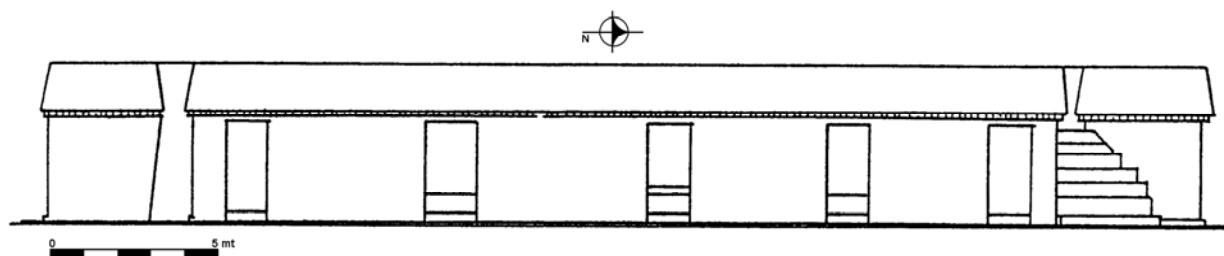
Figura 7 Estructura 5C-45-4A: elevación
