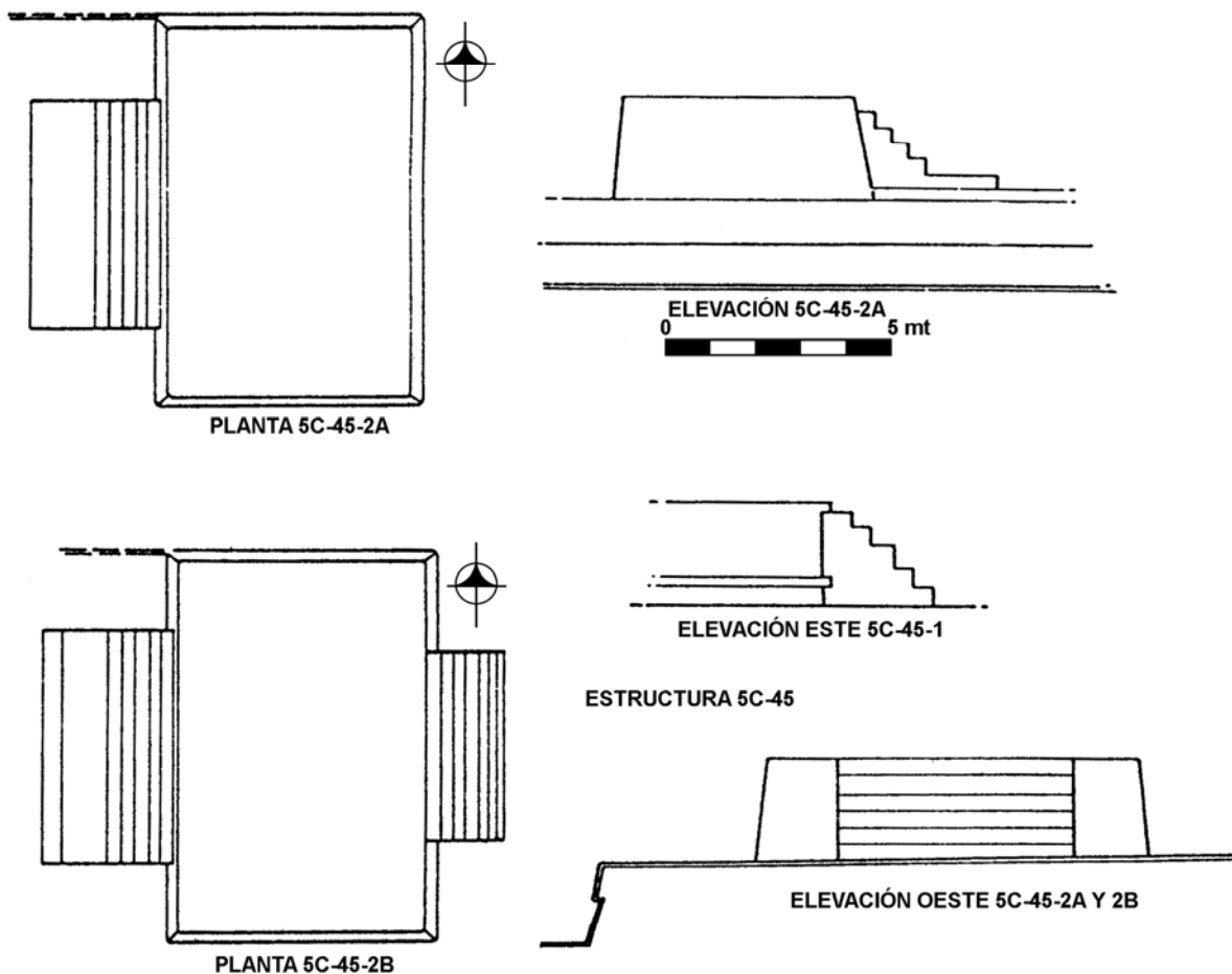
Figura 4 Estructura 5C-45-1, 2A y 2B: planta y perfil
