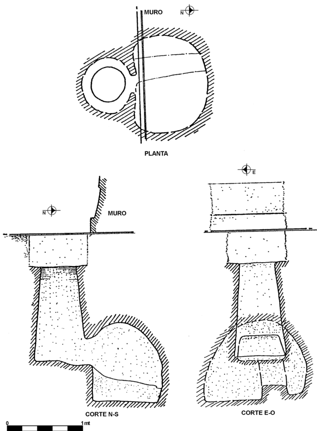
Figura 23 Perfiles de chultun bajo Estructura 5C-46
