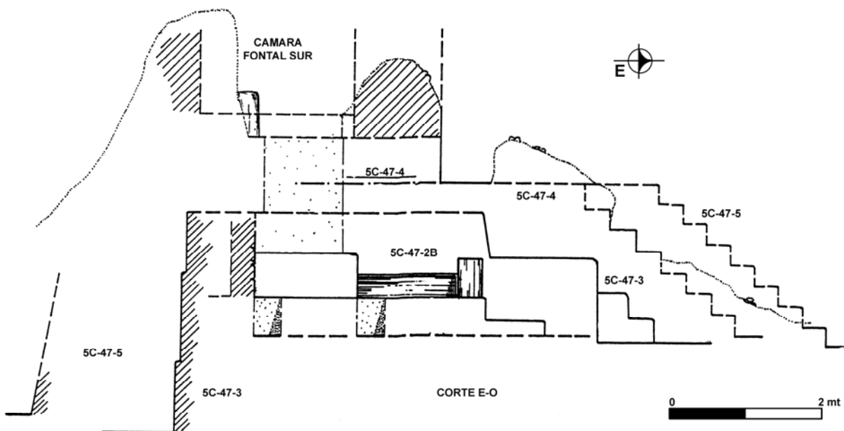
Figura 29 Estructura 5C-47: corte este-oeste general
