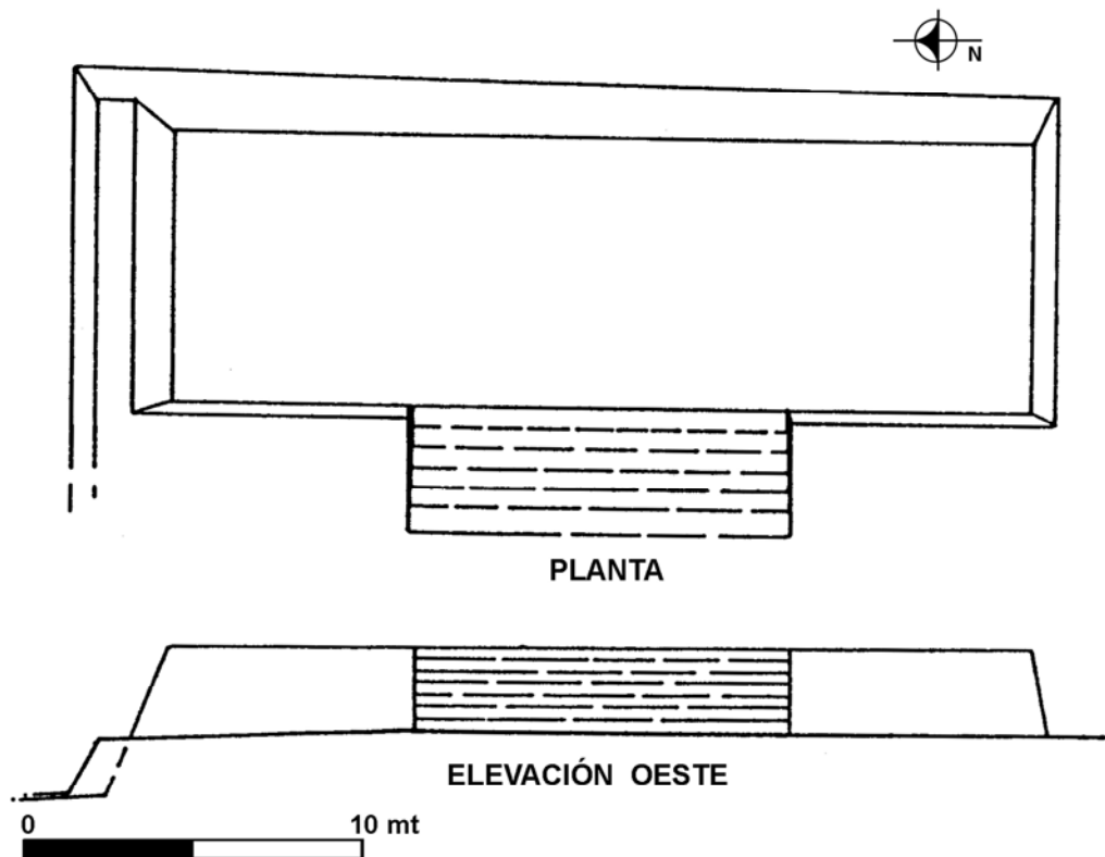
Figura 5 Estructura 5C-45-3: planta y elevación
