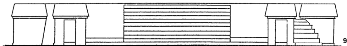
Figura 8 y 9 Estructura 5C-45-4B: planta y elevación
