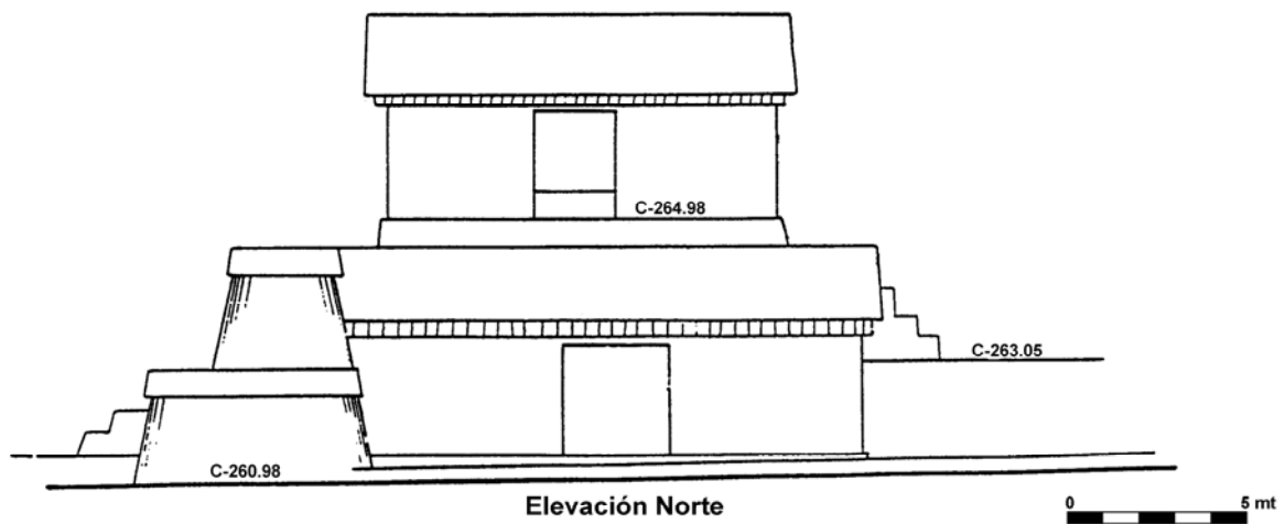
Figura 12 Estructura 5C-45-5A: elevación
