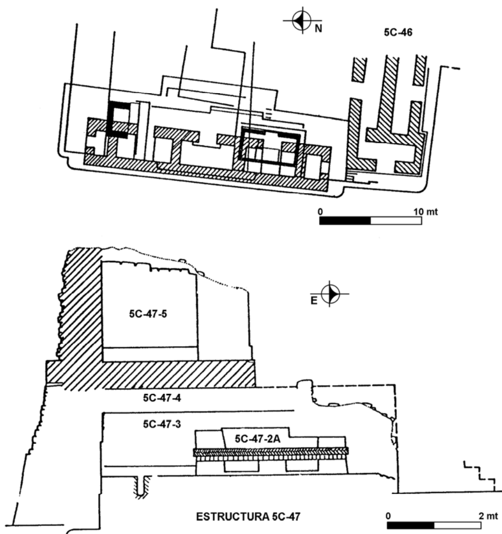
Figura 28 Estructura 5C-47: planta y corte este-oeste en sector de banca decorada
