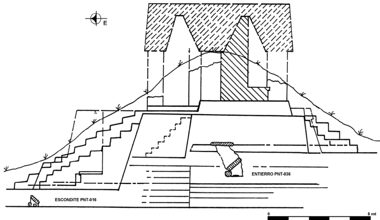
Figura 3 Corte este-oeste de la Estructura 5C-45
