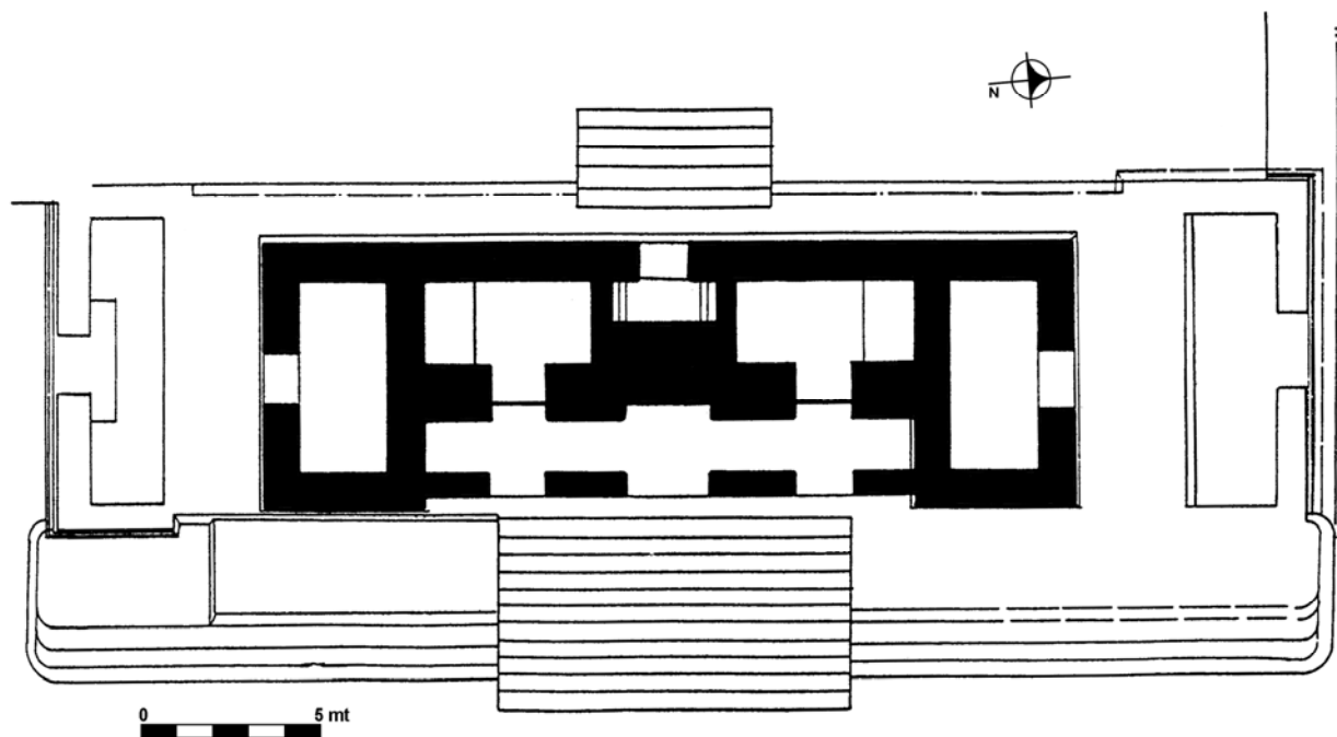
Figura 11 Estructura 5C-45-5B: planta
