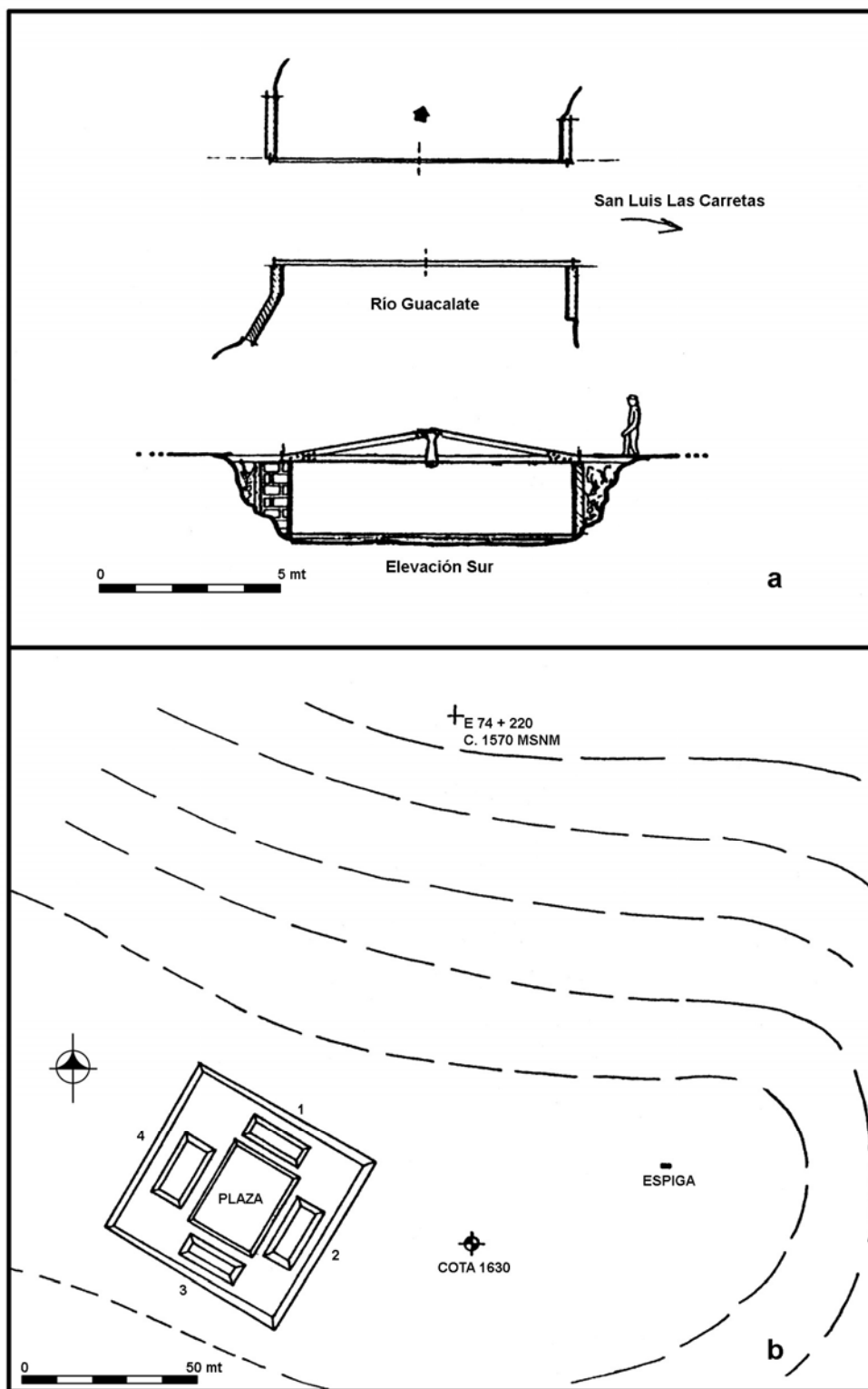
Figura 4a) Planta y elevación del puente sobre el río Guacalate; b) Planta del sitio arqueológico Los Venados (Dibujo: Paulino Morales)
