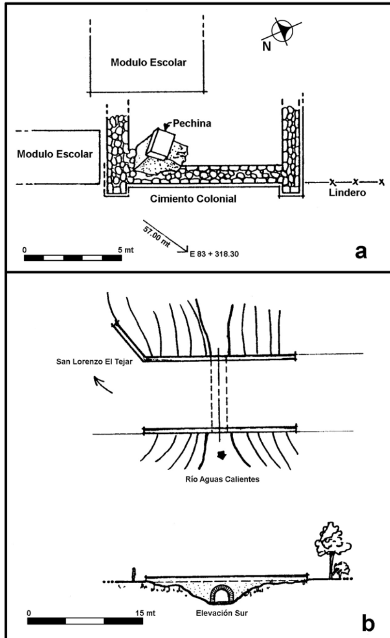
Figura 3a) Plano de cimentación de la iglesia colonial de San Lorenzo el Tejar; b) Planta y elevación del puente sobre el río Aguas Calientes (Dibujo: Paulino Morales)
