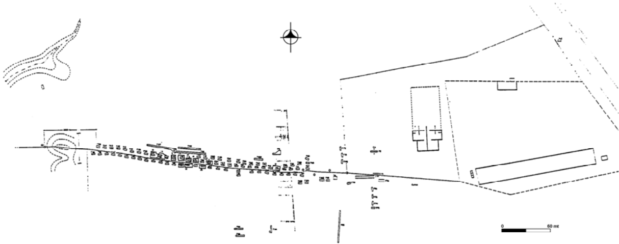
Figura 5 Planta de investigación, Destacamento Militar de Belén
