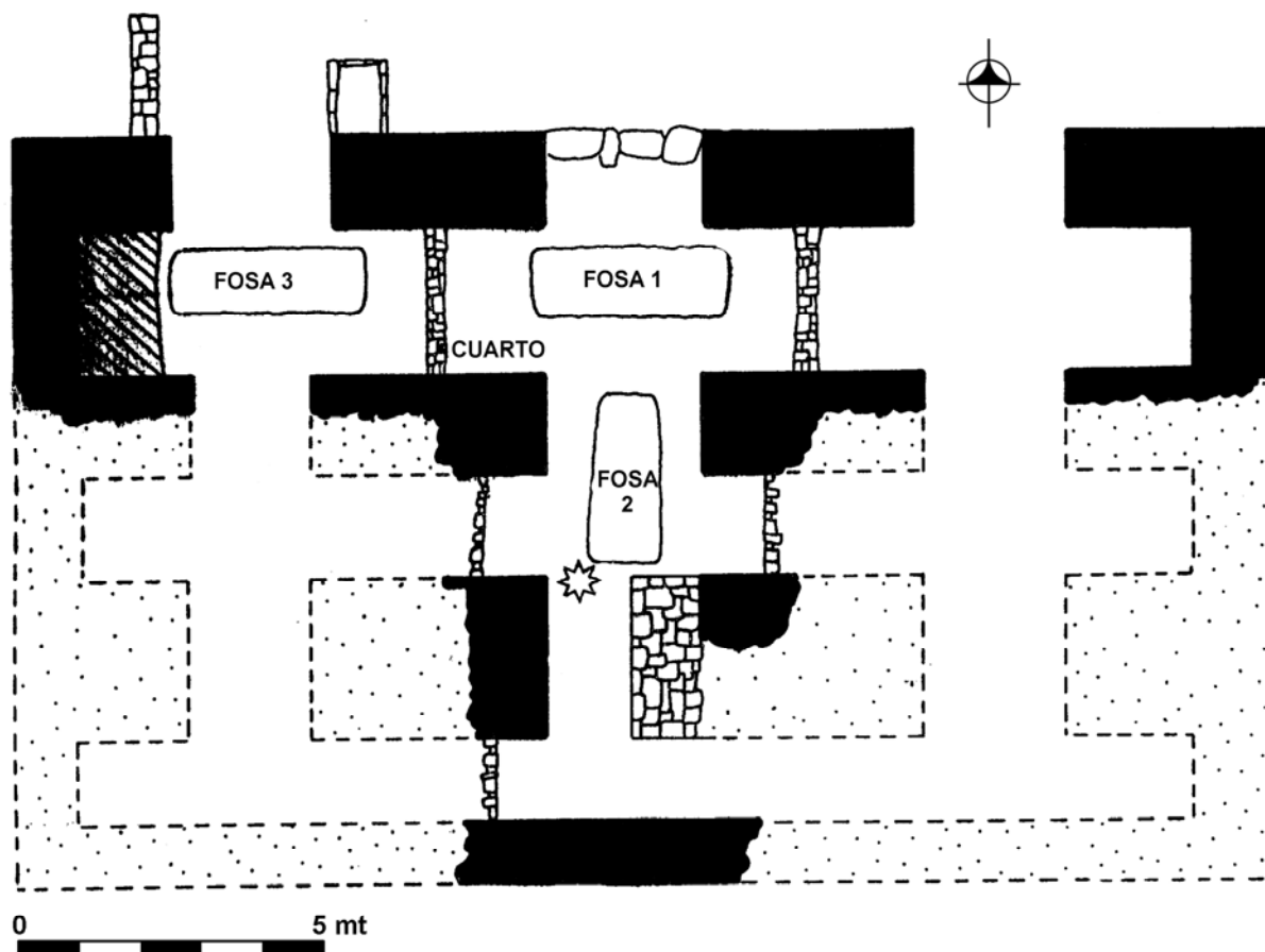
Figura 2 Dibujo en planta del Edificio IIB de Calakmul, Campeche, realizado por Sophia Pincemin (1988), mostrando la ubicación de las fosas correspondiente a los Entierros II-3, II-4 y II-5
