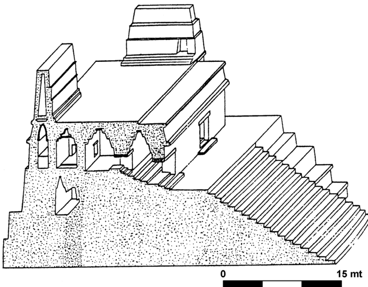
Figura 6 Dibujo del corte transversal de la Estructura III realizado por Sophia Pincemin (1994), mostrando la ubicación de la tumba
