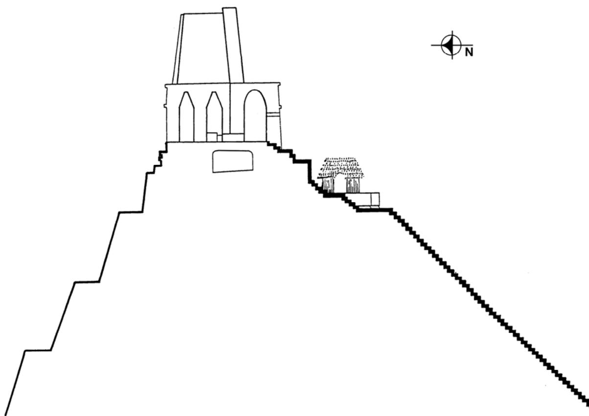
Figura 4 Dibujo del corte transversal de la cuarta etapa constructiva de la Estructura VII realizado por Aída Amine Casanova y Ma. del Rosario Domínguez, mostrando la ubicación del entierro (Domínguez 1993)
