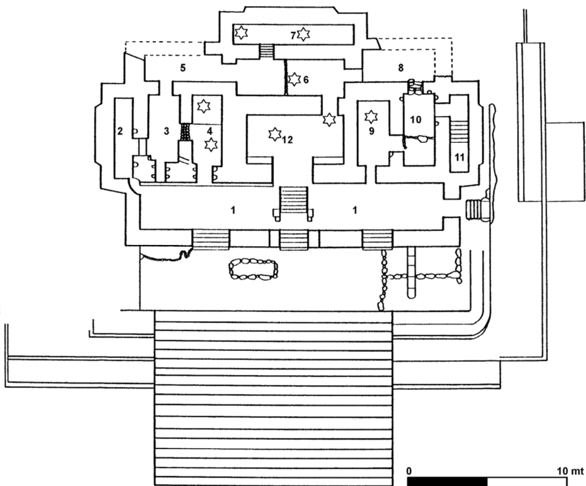
Figura 3 Dibujo en planta de la Estructura III de Calakmul realizado por Álvarez y Armijo (1989-1990), basado en Ruppert y Denison de Carnegie Institution, mostrando la ubicación de los entierros localizados en dicha estructura
