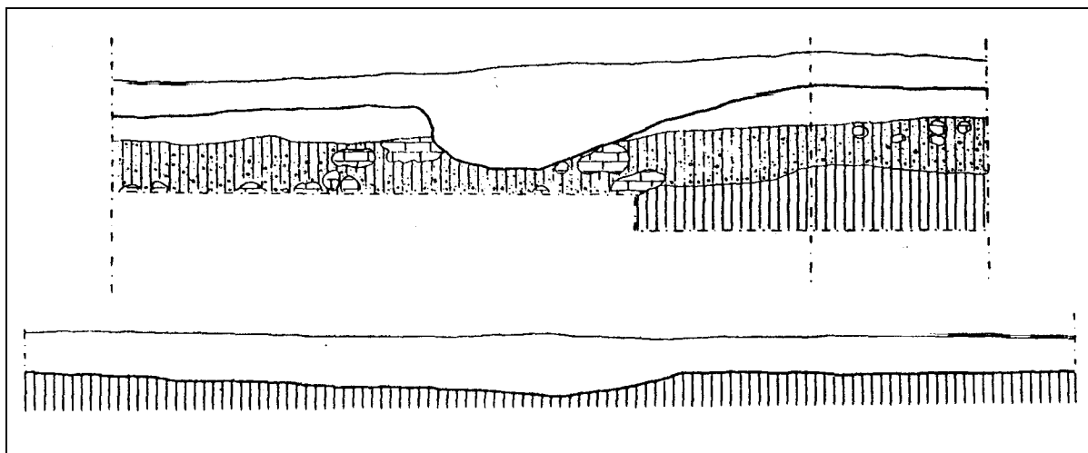
Figura 17 Perfil oeste, Unidad KJM 3B-69 (arriba) y perfil este, KJM 3B-201, Canal Mirador
