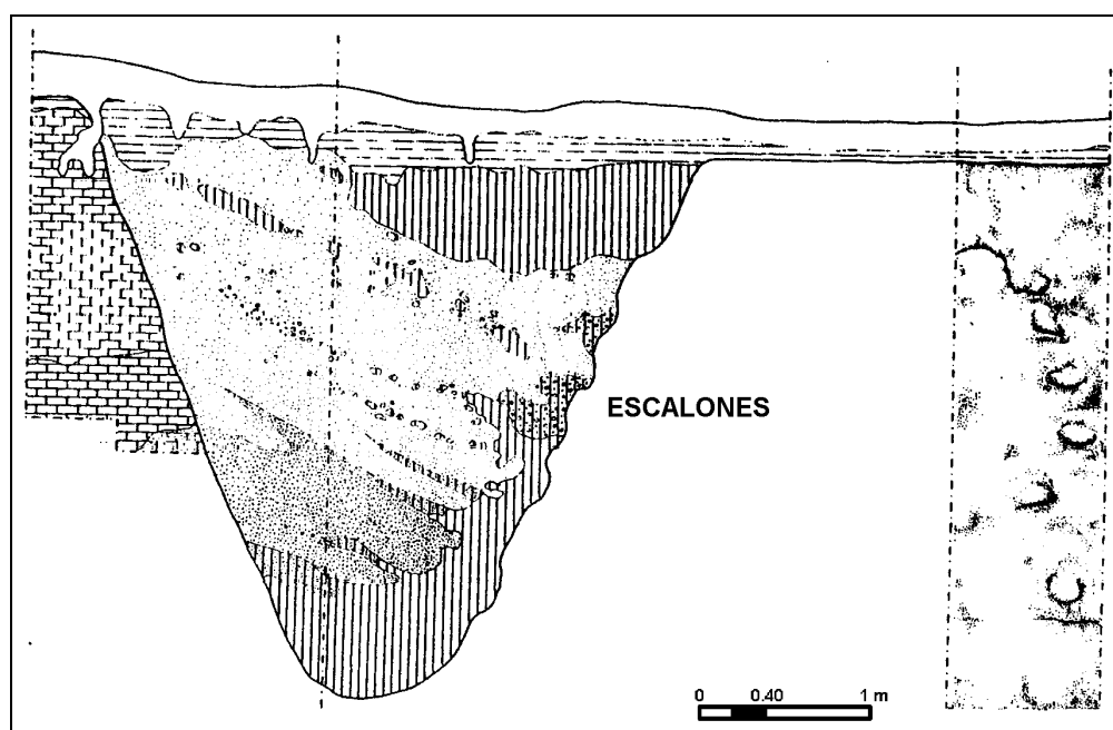
Figura 11 Perfil norte, Unidades KJM 3A-1, 3A-16, Canal Miraflores
