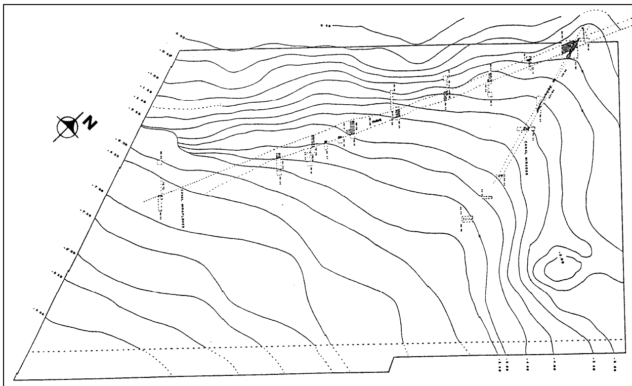
Figura 4 Mapa topográfico del Sector 3, con canales Miraflores y Mirador, Proyecto Kaminaljuyu Miraflores II
