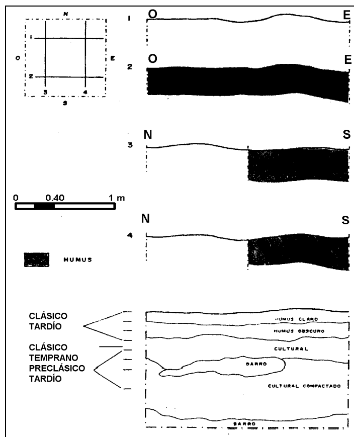
Figura 7 Perfiles, Unidad KJM 3B-72 (nótese la superficie mostrando surcos de cultivo)
