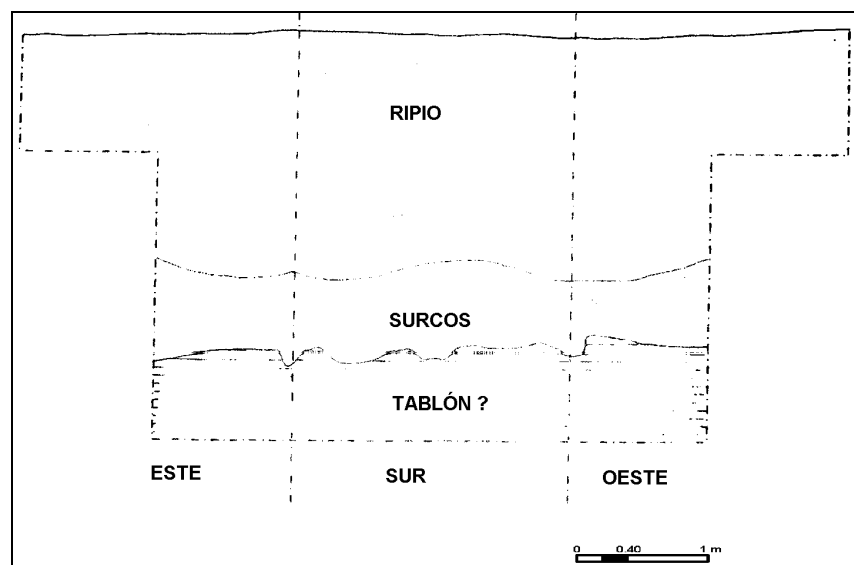
Figura 8 Perfil este-suroeste, Unidad KJM 3B-99 (nótese la superficie mostrando surcos de cultivo posible tablón)
