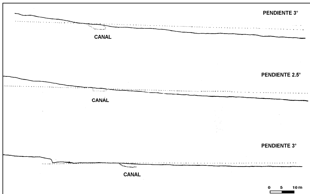
Figura 6 Perfil este-oeste del Sector 3, con la ubicación del canal Miraflores y la pendiente natural del terreno
