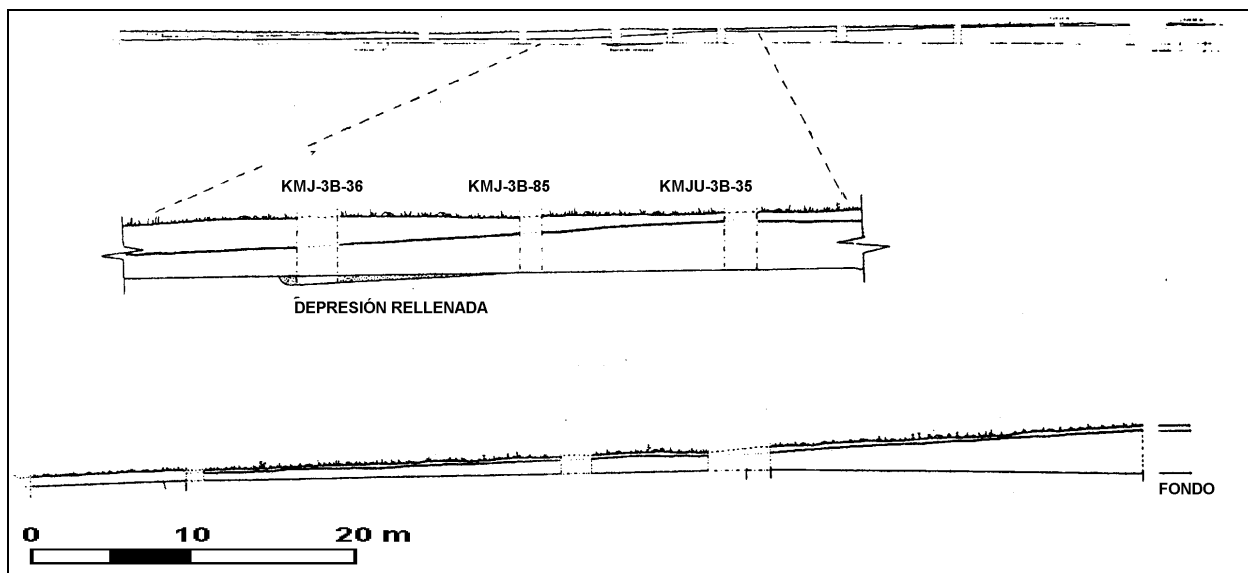
Figura 5 Perfil norte-sur de los canales Miraflores (arriba) y Mirador (abajo)
