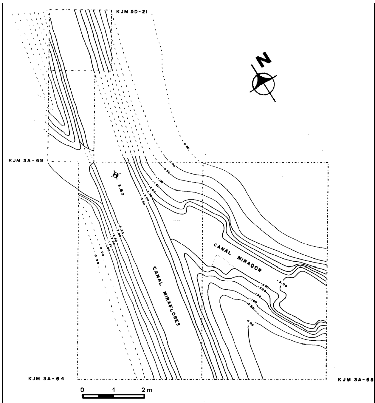
Figura 15 Detalle topográfico de la intersección de los canales Mirador y Miraflores
