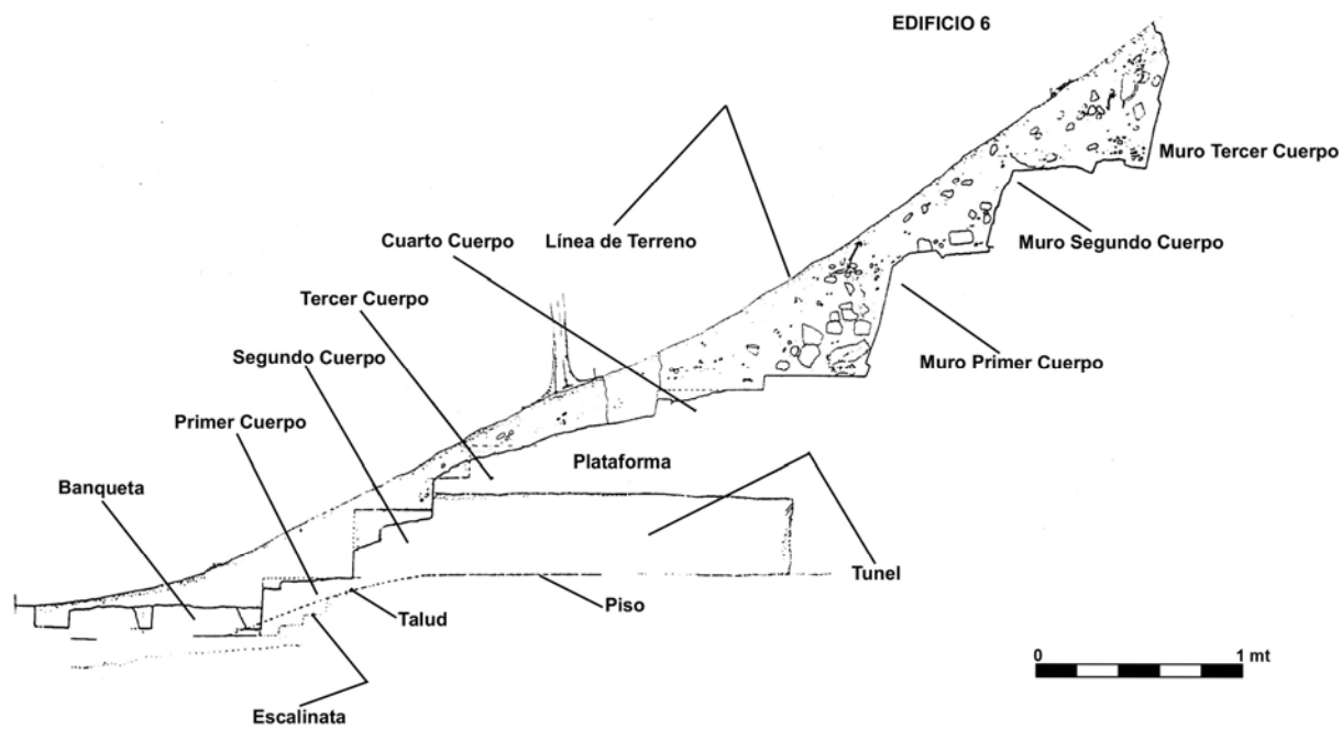
Figura 10 Corte este-oeste de Edificio 6
