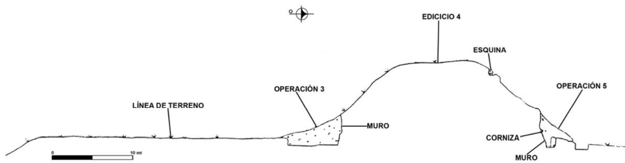
Figura 7 Perfil este-oeste de Edificio 4
