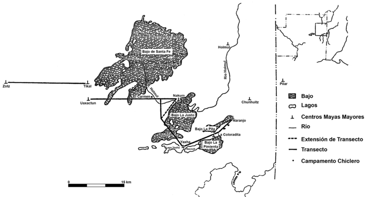
Figura 3 Mapa de bajos Santa Fe, La Justa y La Pimienta
