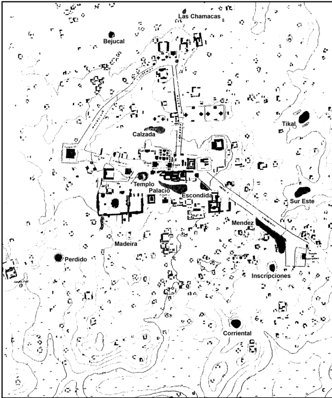
Figura 1 Ubicación de las aguadas de Tikal
