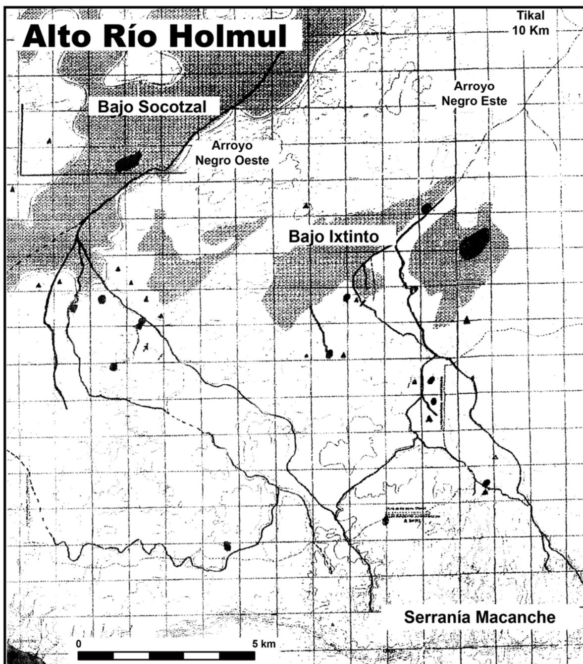
Figura 4 Mapa de bajos Socotzal e Ixtinto
