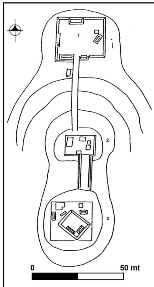
Figura 4 a) Planta de distribución de grupos de Chiquibul 1; b) Planta del área central de Chiquibul 1
