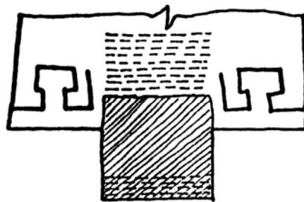
Figura 7 Planta del tercer estadio constructivo
