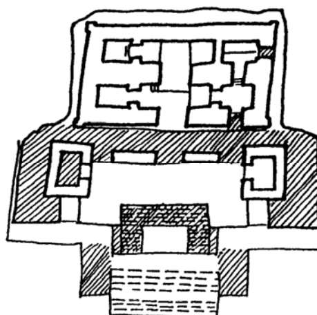
Figura 11 Planta del séptimo estadio constructivo
