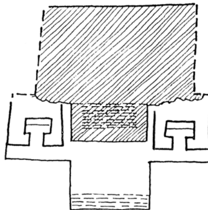
Figura 8 Planta del cuarto estadio constructivo
