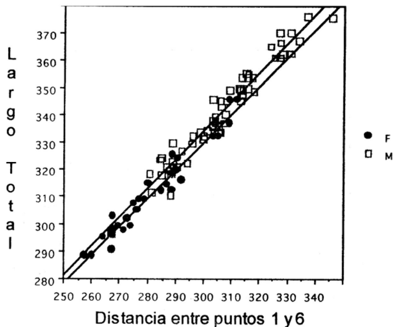
Figura 1 Relación entre el largo total de la tibia y la distancia entre dos puntos en ella, en 100 esqueletos forenses indígenas
