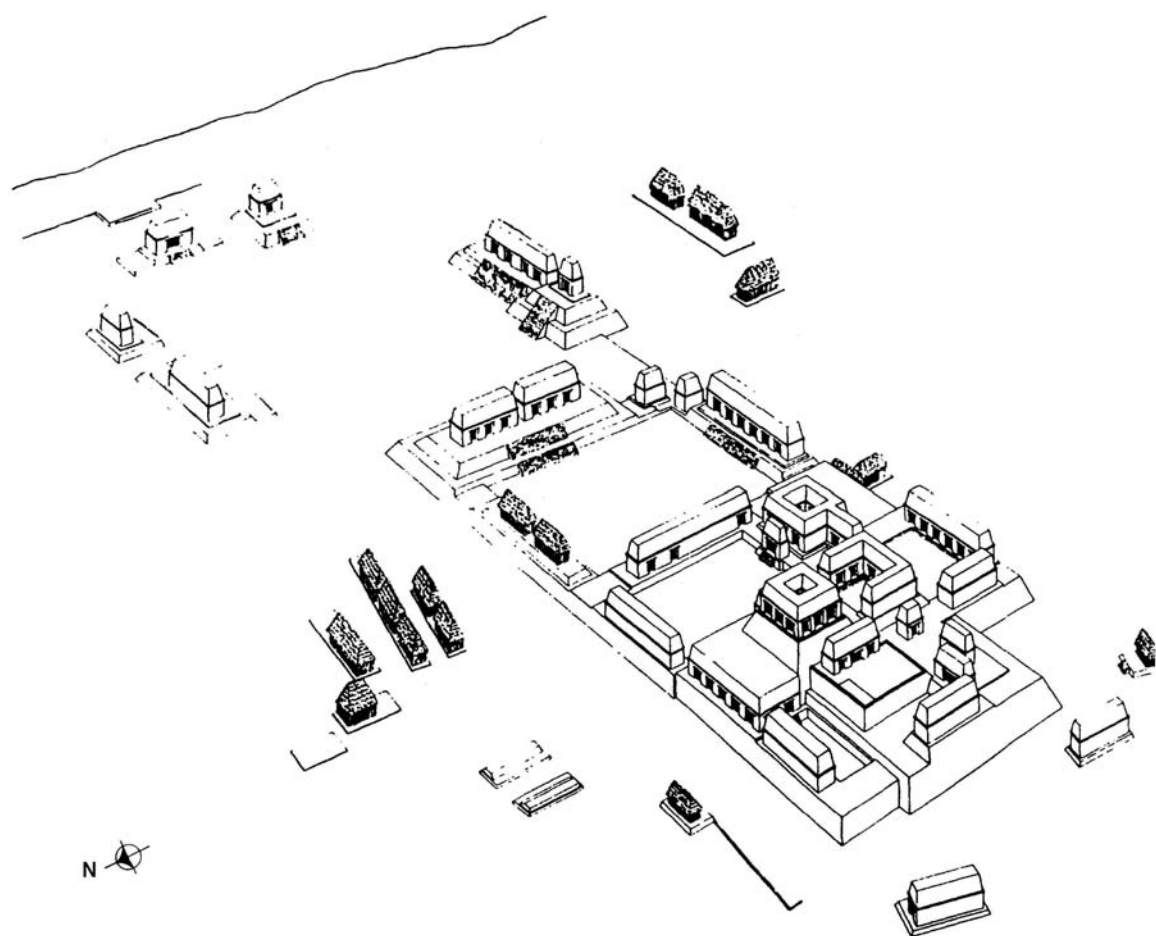
Figura 8 Vista reconstructiva del Palacio de Cancun (dibujo preliminar por L.F. Luin)
