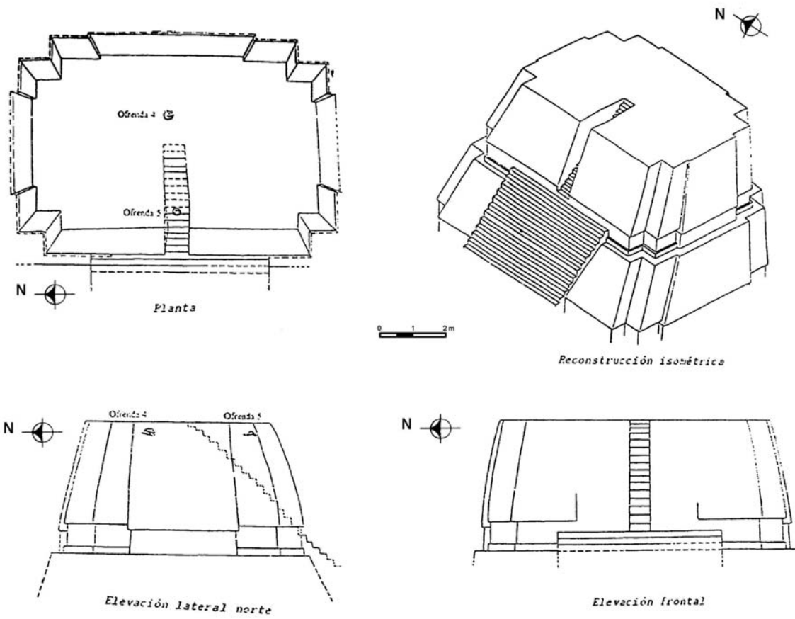
Figura 7 Planta de Chultun 7B-1
