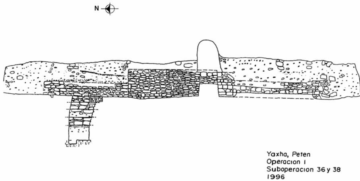
Figura 5 Elevación de la fachada oeste del Edificio 216 Sub-1 de Yaxha
