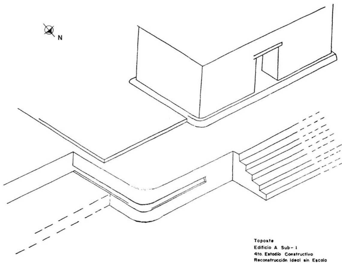
Figura 11 Reconstrucción ideal del Edificio A Sub-1 de Topoxte
