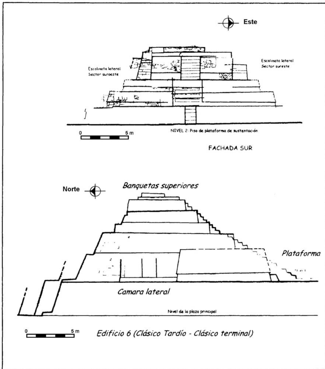
Figura 9 Fachada sur y oeste del Edificio 6
