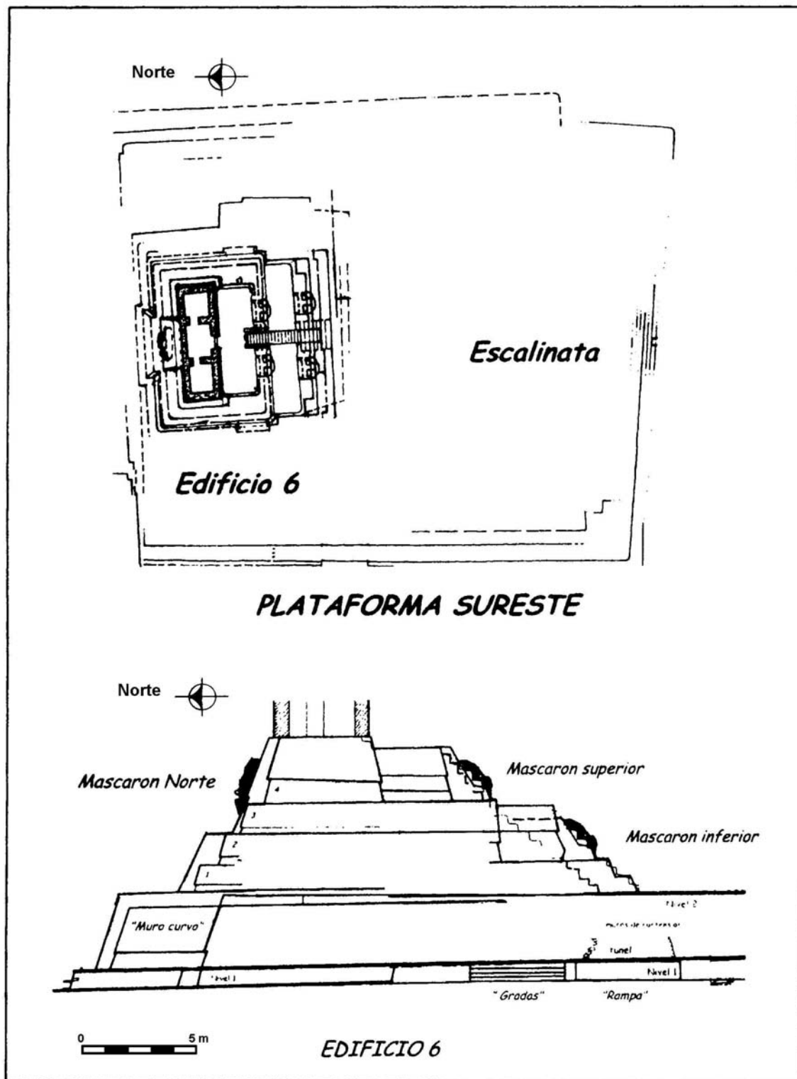
Figura 7 Edificio 6 y ubicación de mascarones
