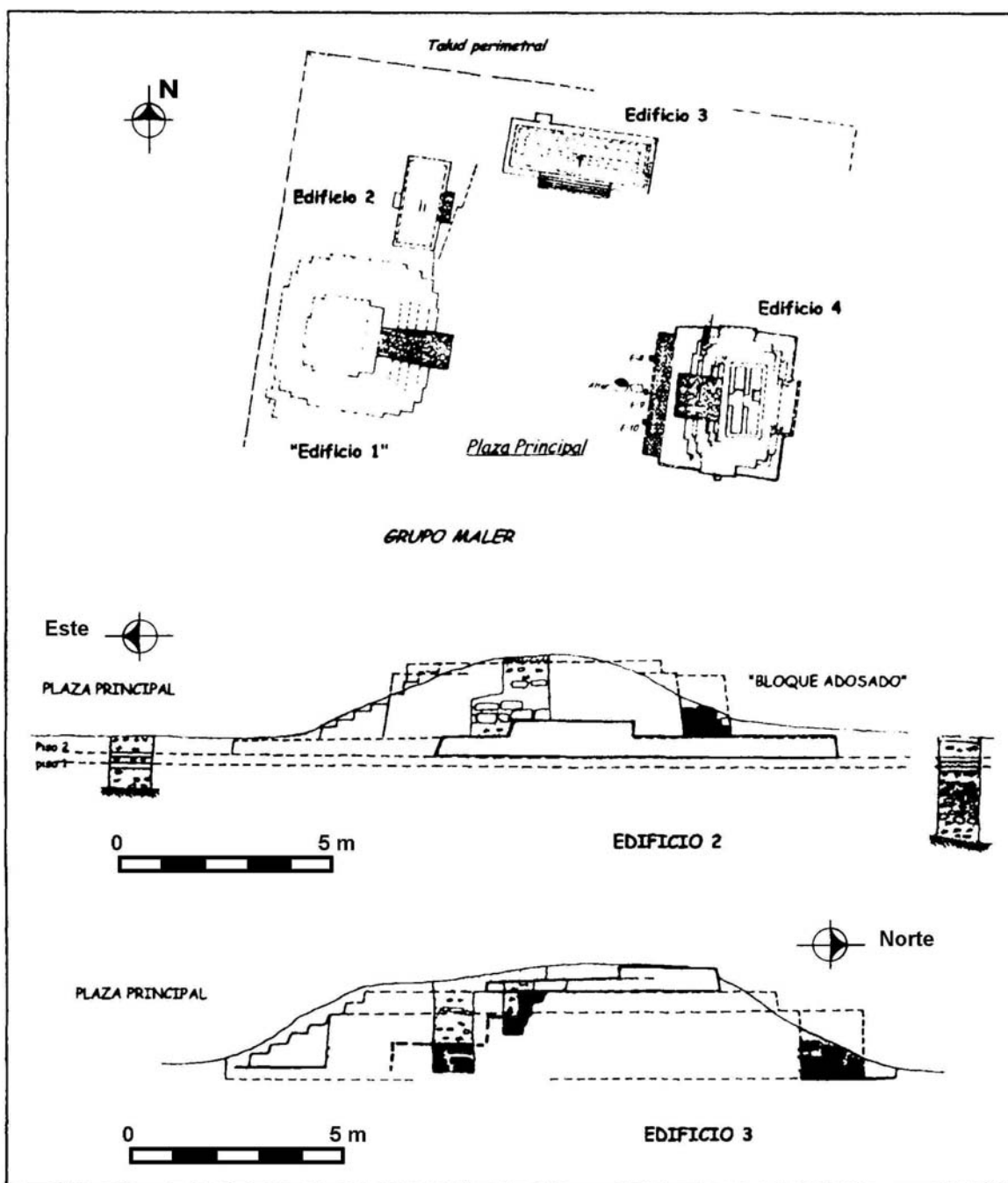
Figura 11 Edificios 2 y 3, Clásico Tardío
