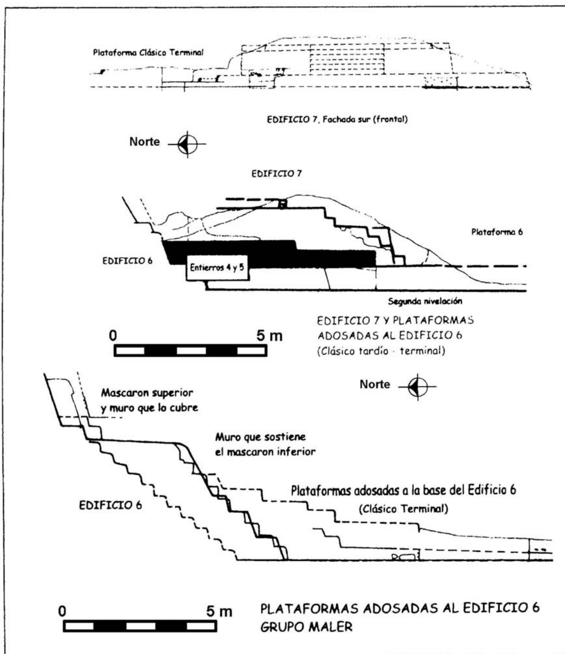
Figura 14 Edificio 7, y plataformas adosada al Edificio 6
