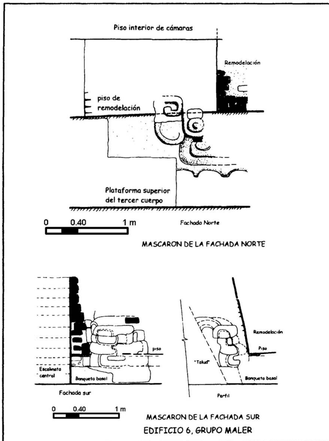
Figura 8 Detalle de mascarones del Edificio 6
