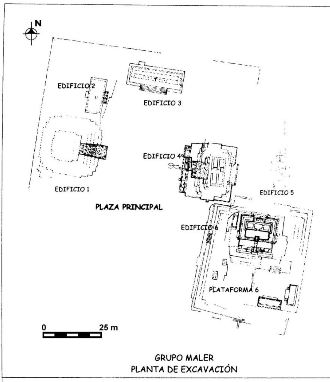
Figura 2 Grupo Maler: planta de excavación
