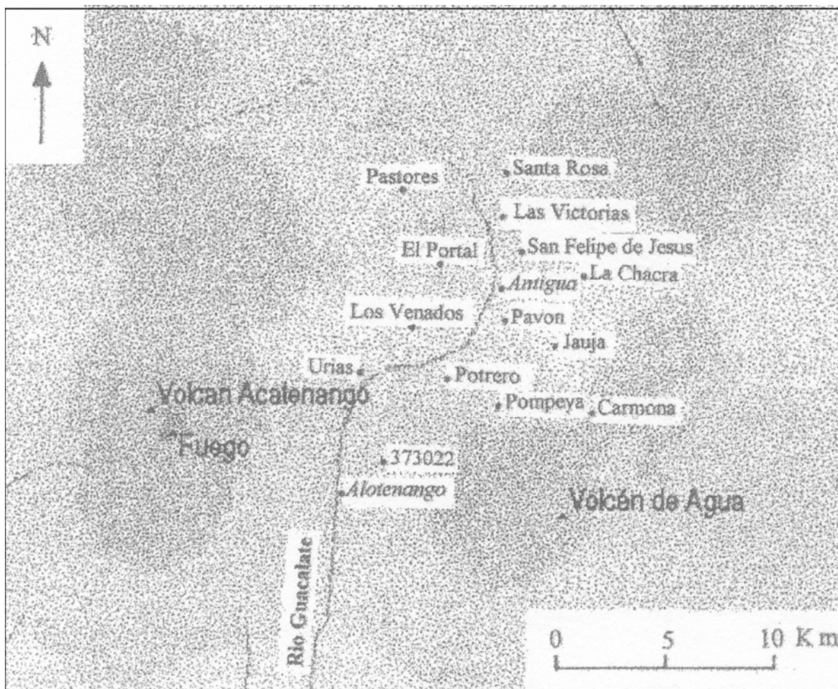
Figura 1 Mapa de la región de Antigua Guatemala, con los sitios mencionados (según el Atlas de Encarta, Microsoft)
