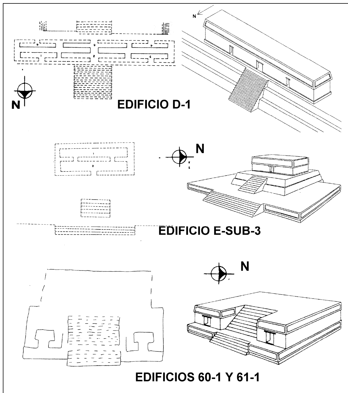
Figura 3 Planta y perspectiva de dos edificios de Nakum
