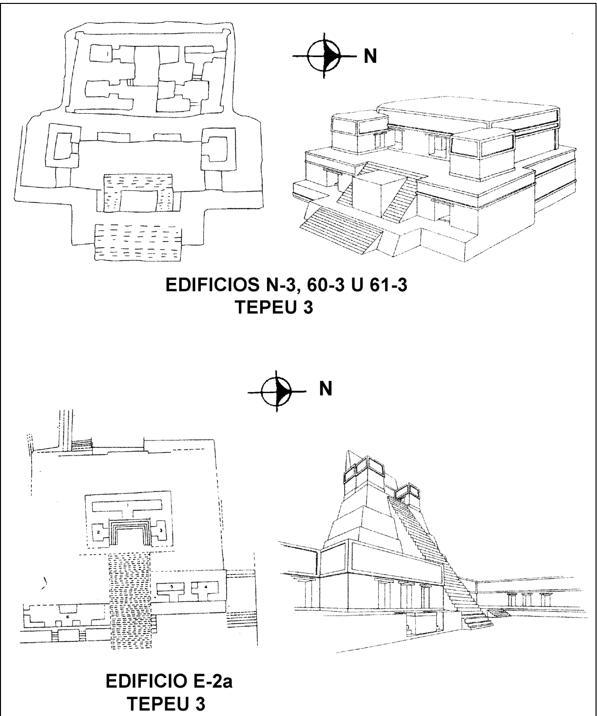
Figura 6 Planta y perspectiva de dos edificios de Nakum
