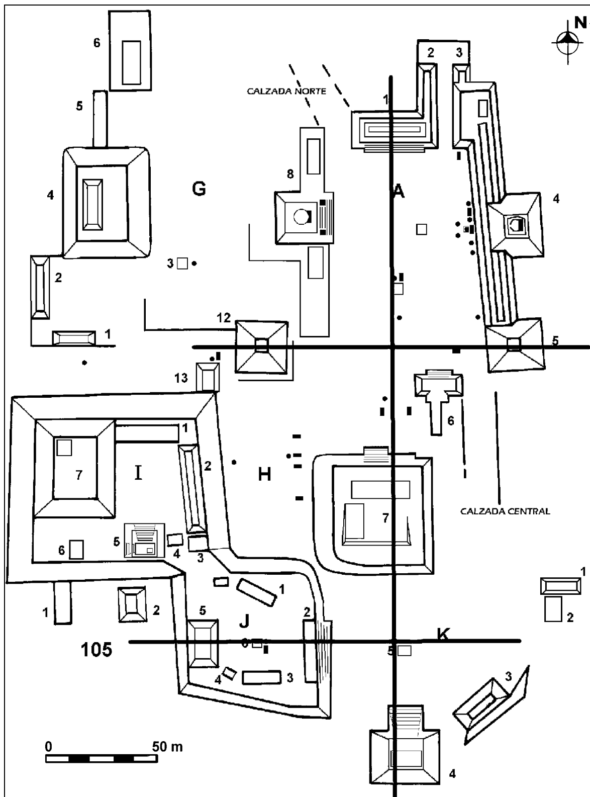
Figura 7 Monumentos marcando ejes constructivos mayores
