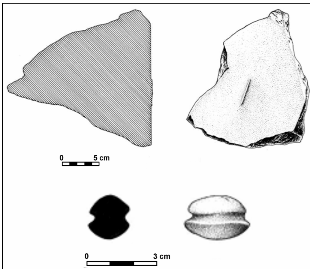
Figura 3 Bloque de jade de 20 libras con marcas de aserrado y una polea para aserrado
