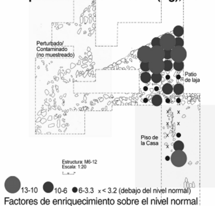
Figura 8 El enriquecimiento de mercurio y oro en el piso de Estructura M6-12
