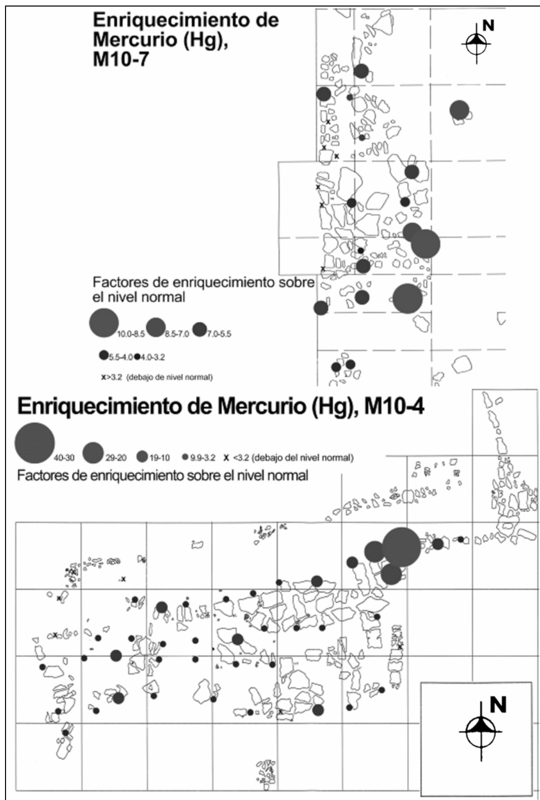
Figura 6 El enriquecimiento de mercurio en los pisos de Estructuras M10-7 y M10-4
