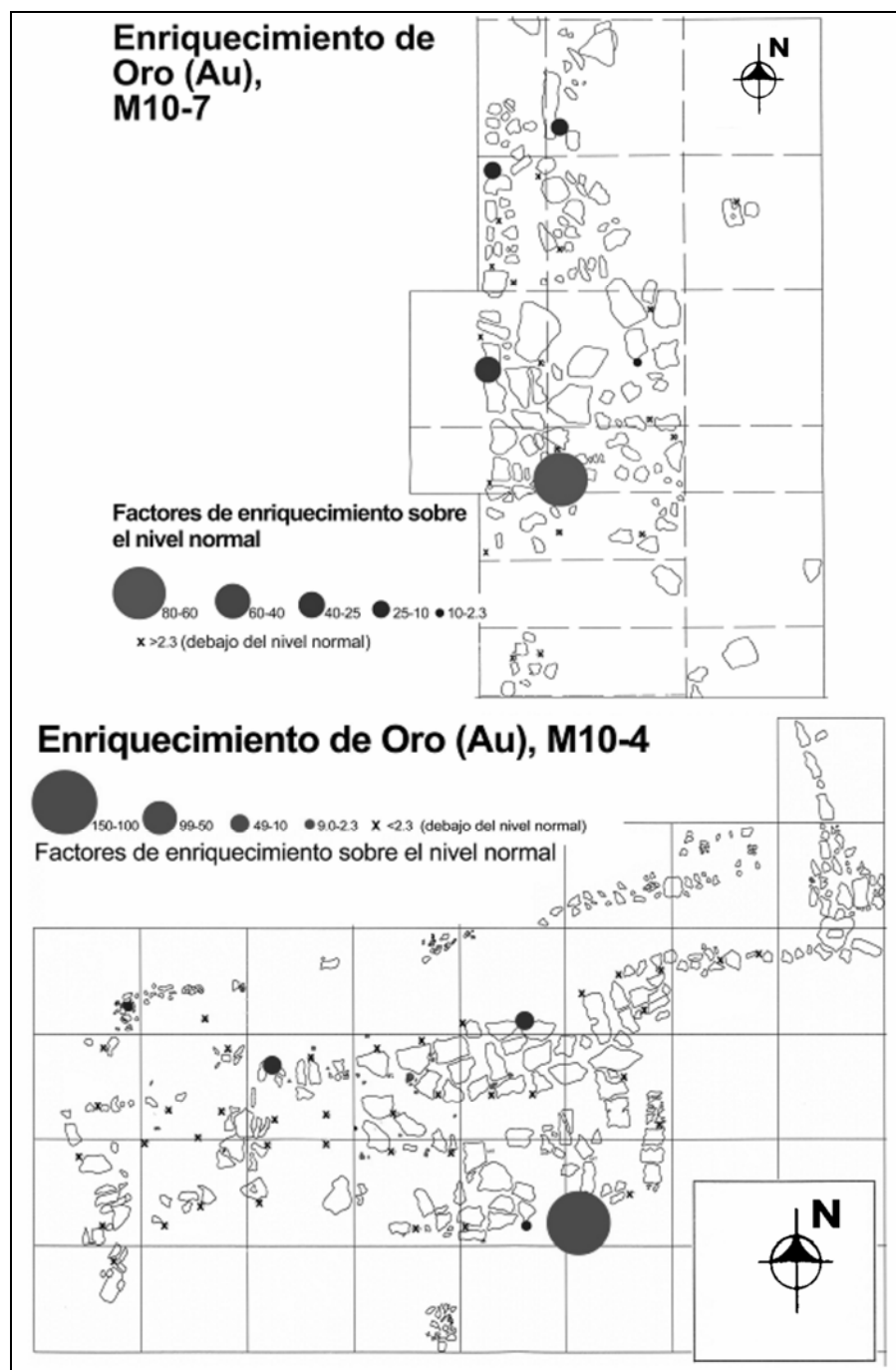
Figura 7 El enriquecimiento de oro en los pisos de Estructuras M10-7 y M10-4
