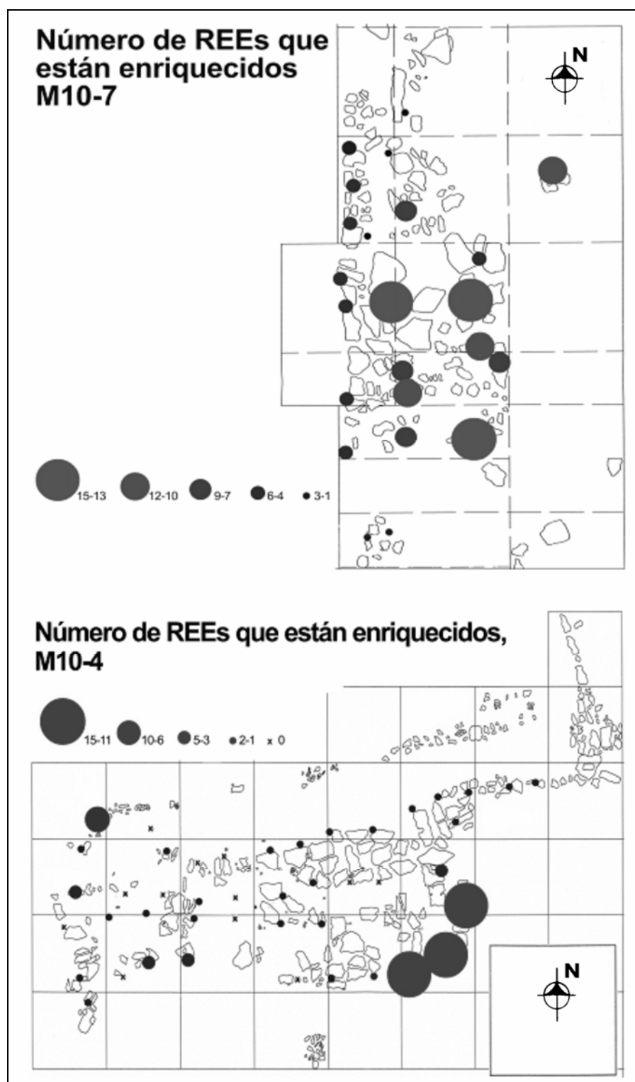
Figura 5 El enriquecimiento de REE ( Rare Earth Elements ) en los pisos de Estructura M10-7 y M10-4
