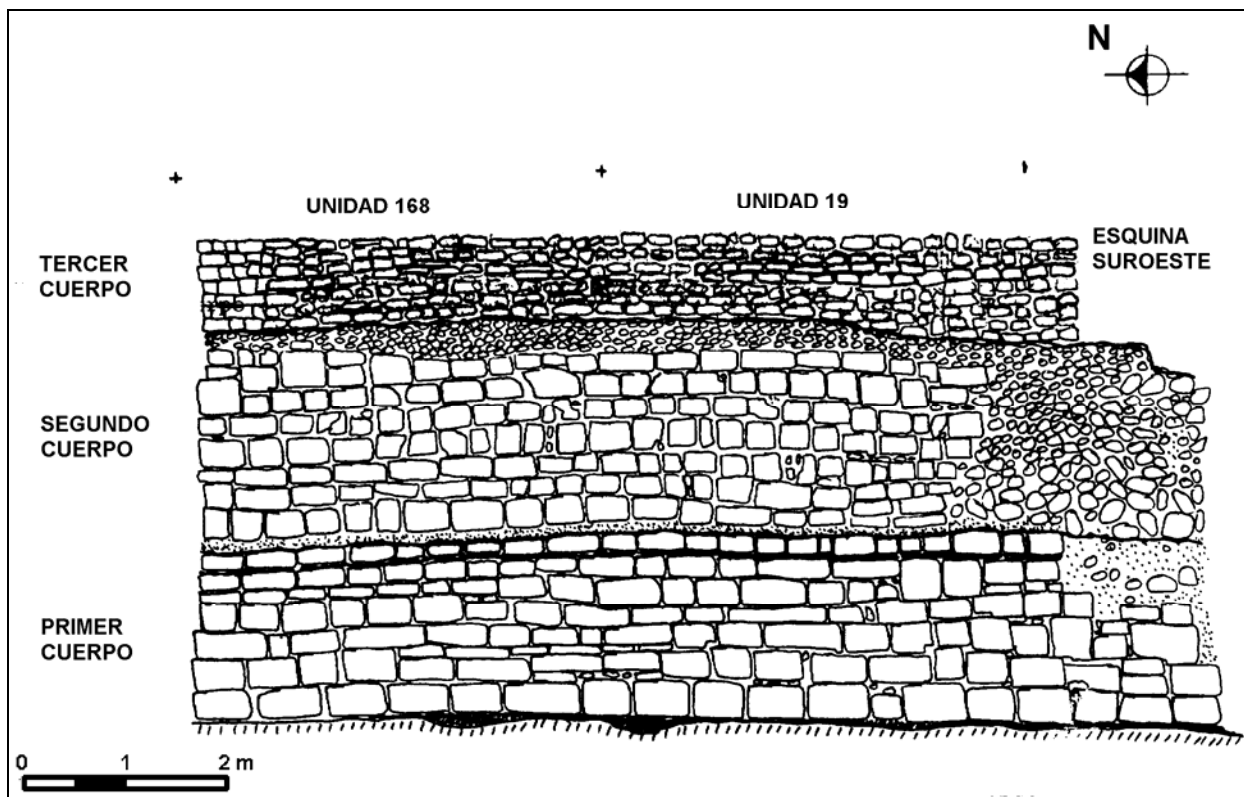
Figura 4 Elevación de la fachada oeste de los cuerpos primero y segundo
