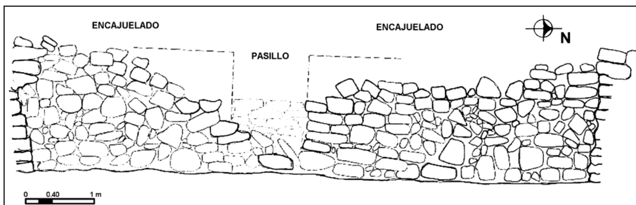
Figura 3 Elevación de la fachada este del encajonado del primer cuerpo
