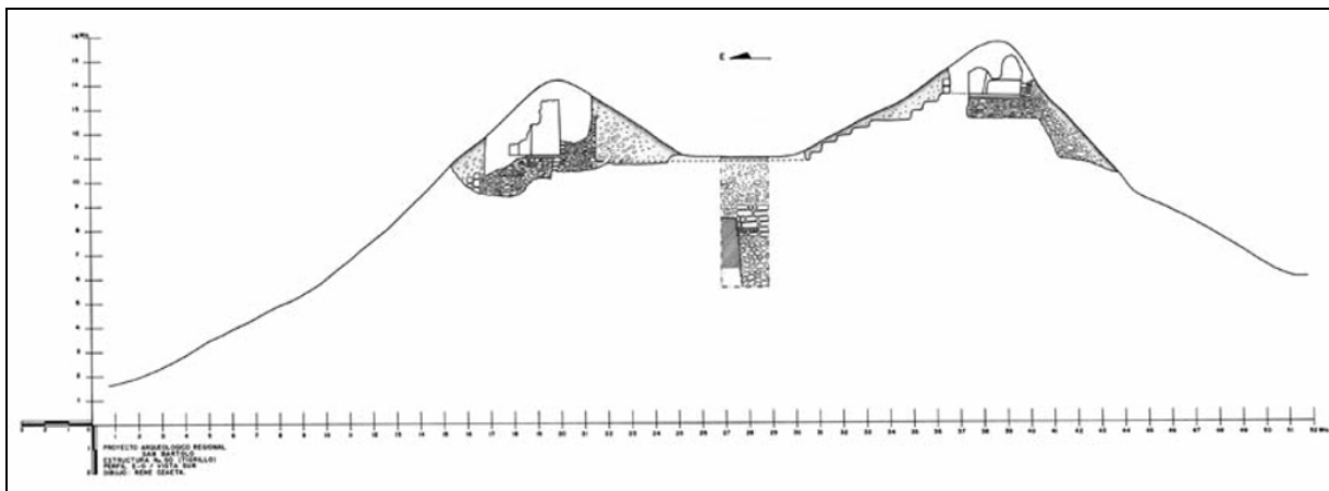
Figura 3 Perfil este-oeste del conjunto palaciego (dibujo de René Ozaeta)
