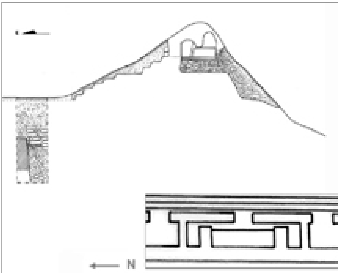
Figura 7 a) Perfil este-oeste del cuarto central con banqueta; b) Plano de la banqueta
