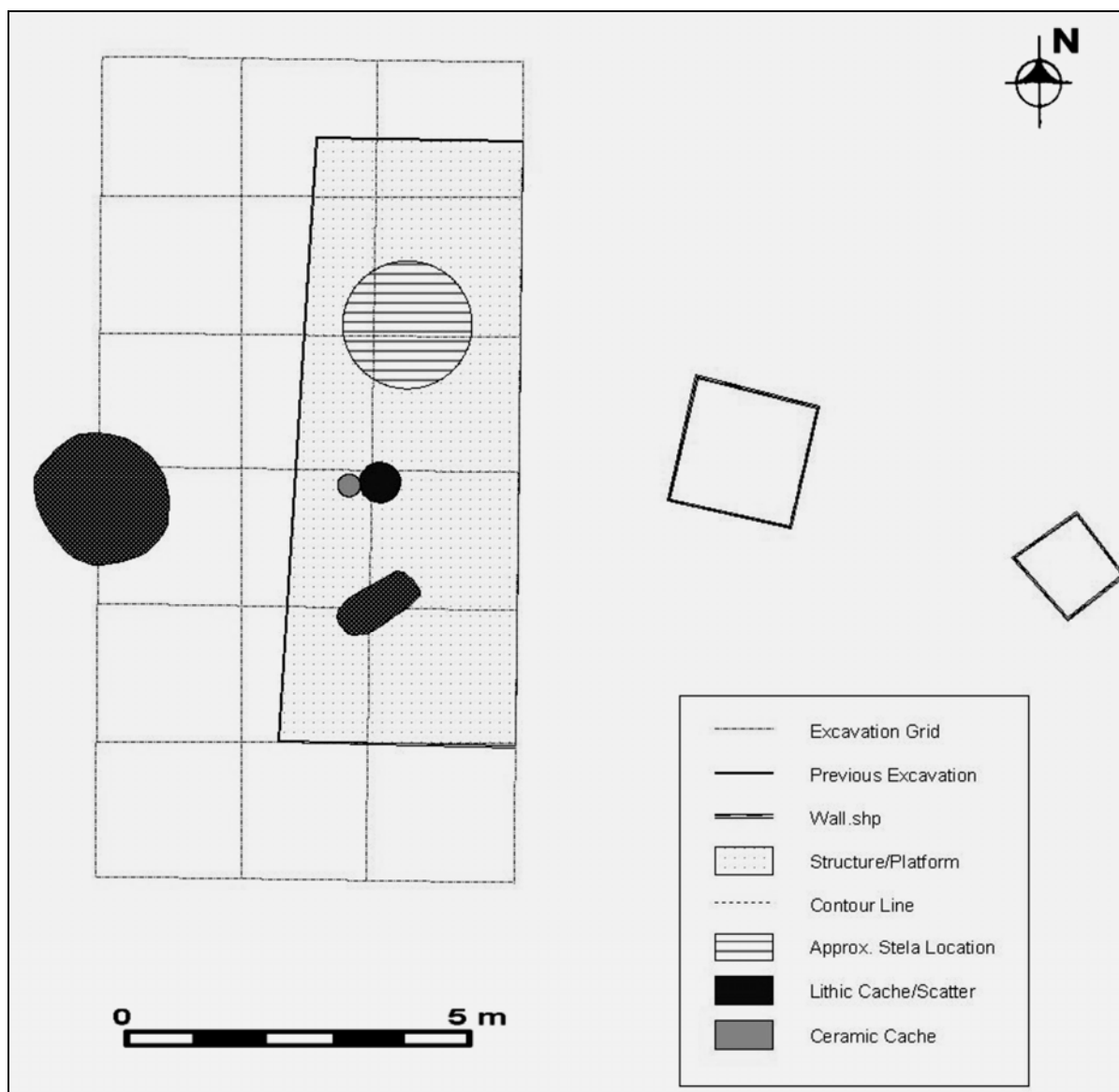
Figura 7 Planta de la posición de monumentos de Tres Islas
