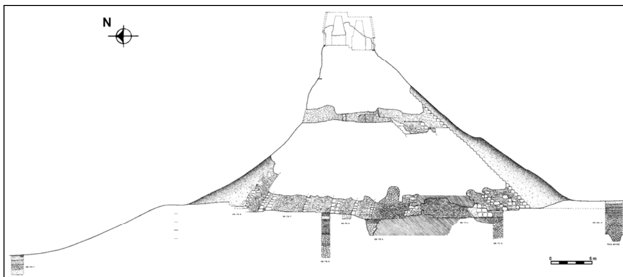
Figura 3 Corte transversal de la Pirámide de Las Ventanas
