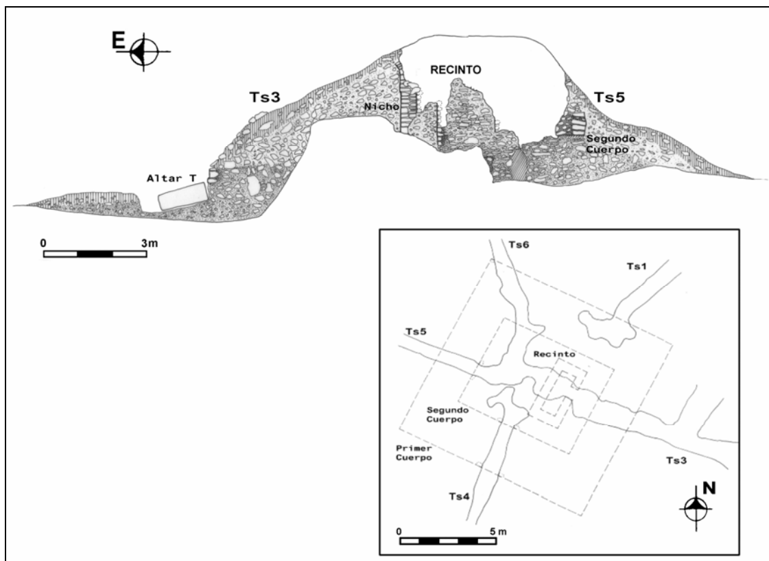
Figura 3 Estructura 4, Planta y perfiles (dibujo Edy Barrios y Véronique Breuil-Martínez)
