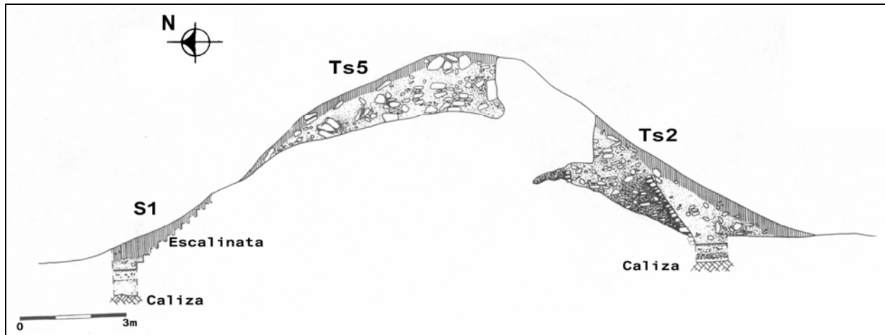
Figura 4 Estructura 55, Planta y perfiles (dibujo Laura Gámez)
