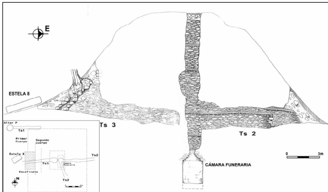
Figura 2 Estructura 2, Planta y perfiles (dibujo Véronique Breuil-Martínez)
