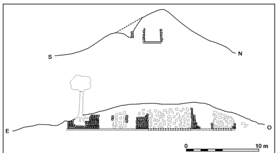
Figura 5 Perfiles de la Estructura 29
