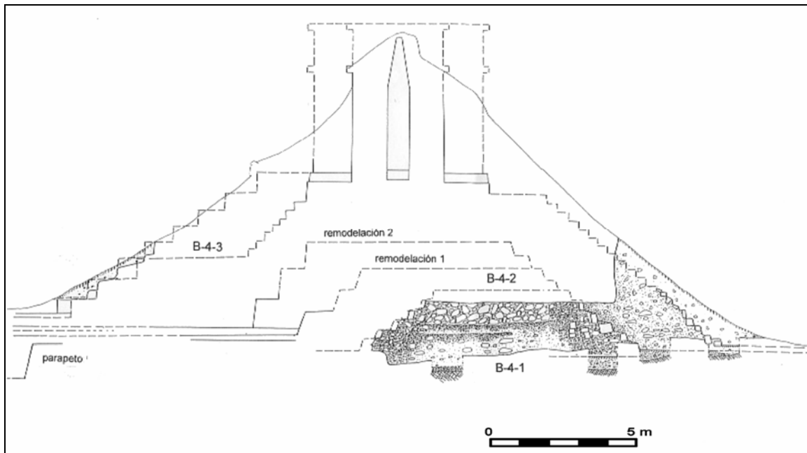
Figura 4 Templo B-4: periodos culturales
