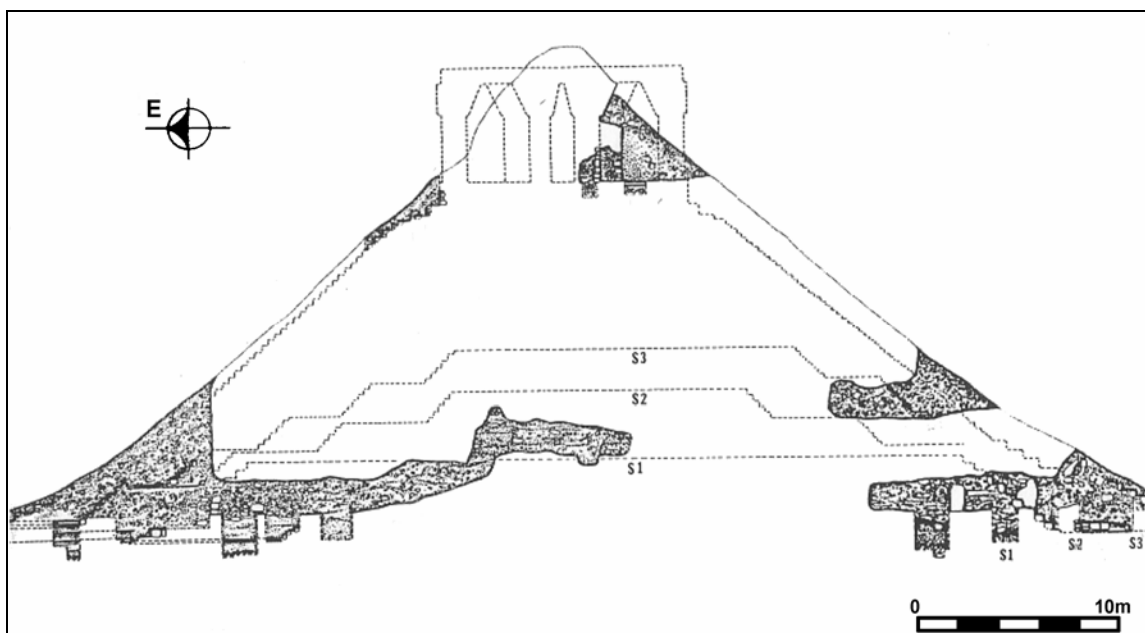
Figura 3 Pirámide B-18: periodos culturales
