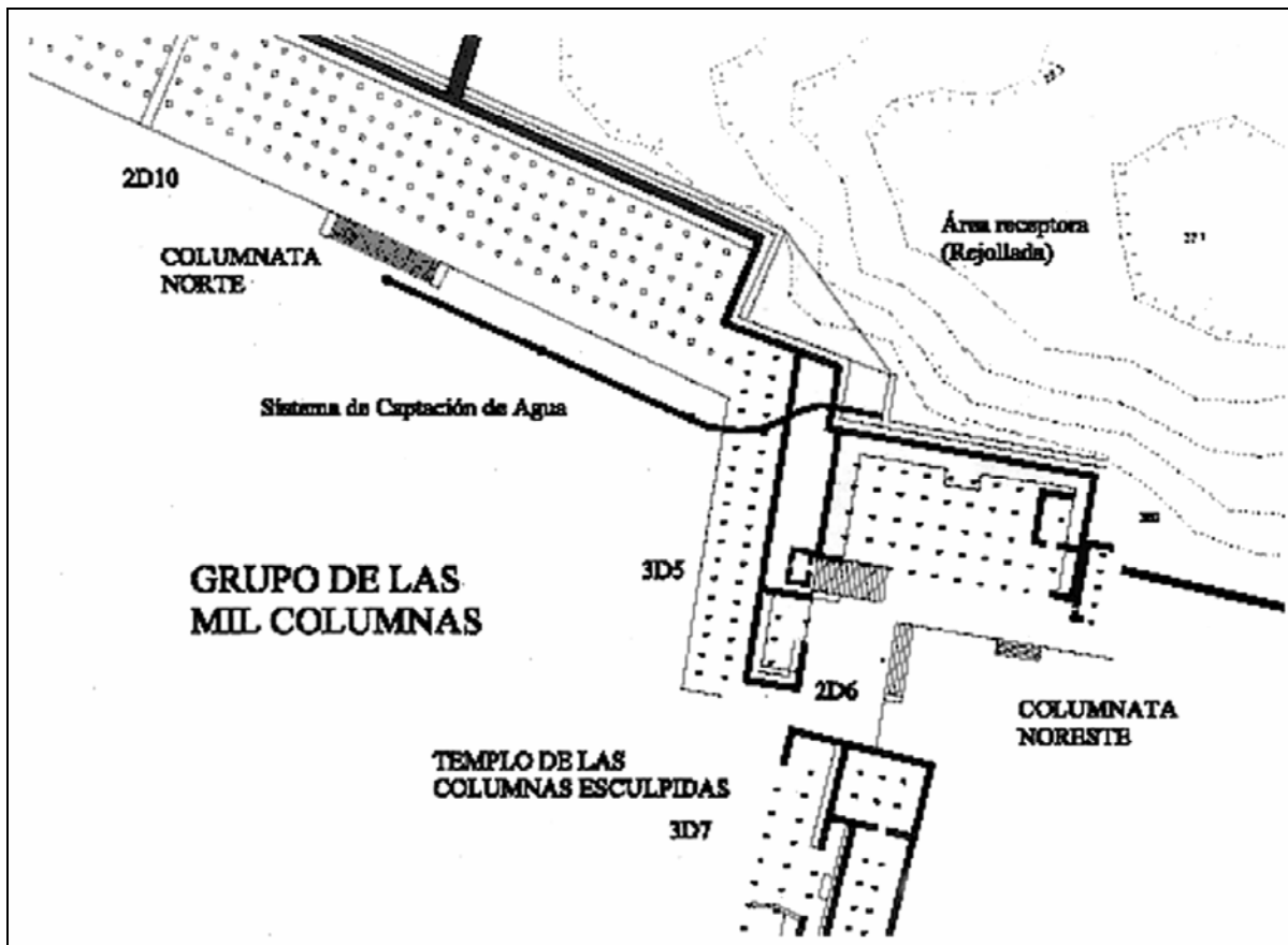
Figura 1 Planta de Grupo de las Mil Columnas
