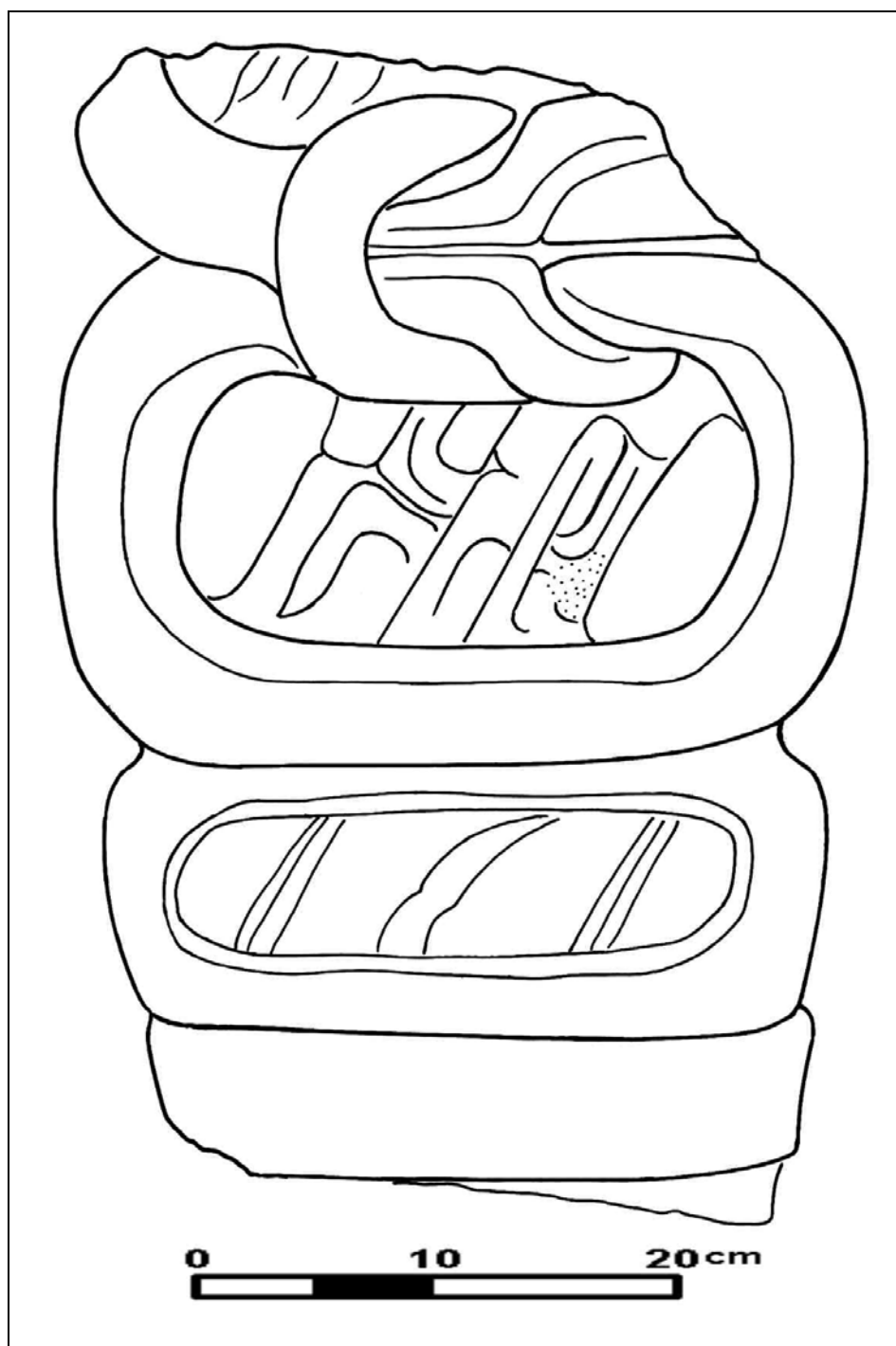
Figura 1 Fragmentos de monumento Preclásico
