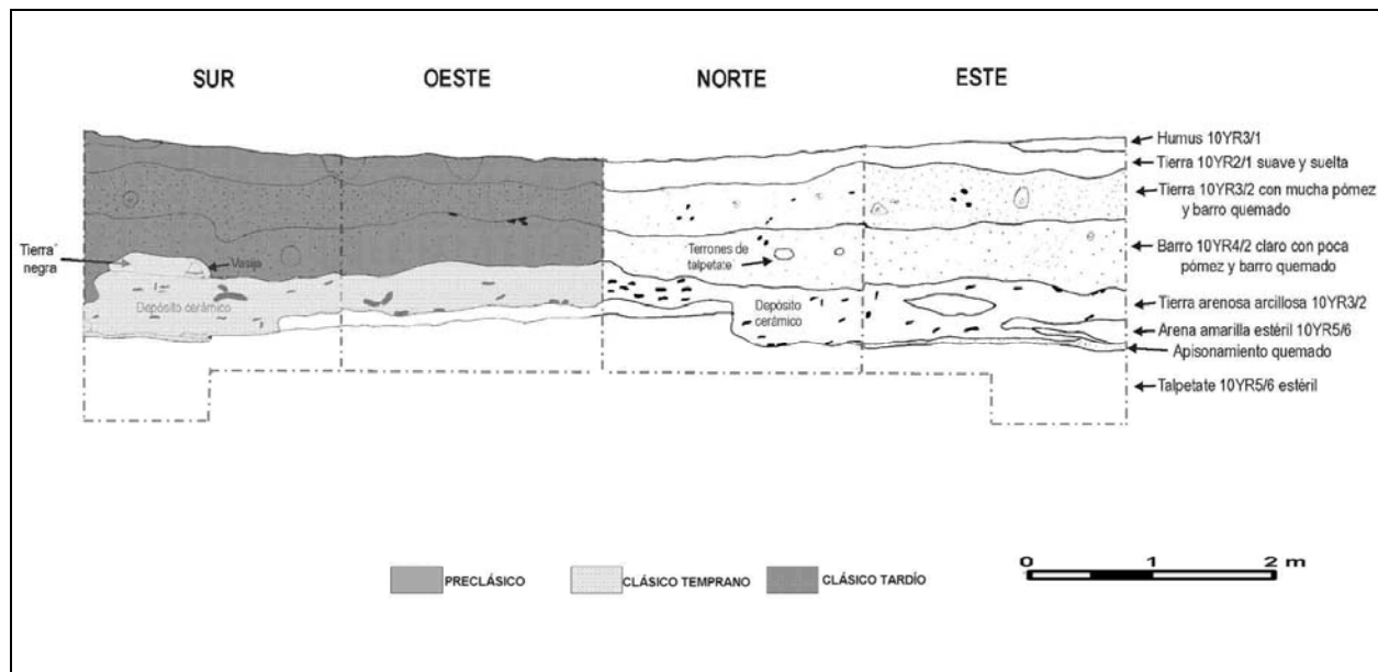
Figura 2 Perfil KJP C6/14
