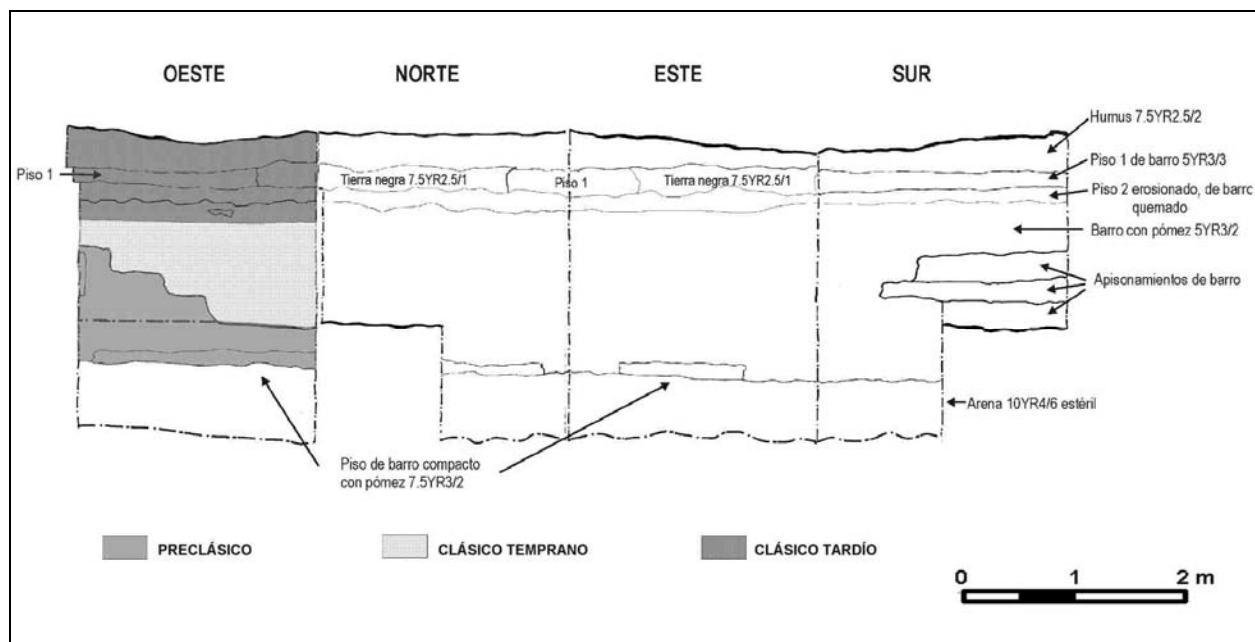
Figura 3 Perfil KJP E9/2
