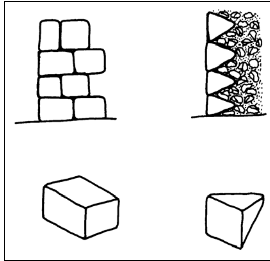
Figura 5 Técnicas constructivas: a) Piedras en saga; b) Piedras de fachada
