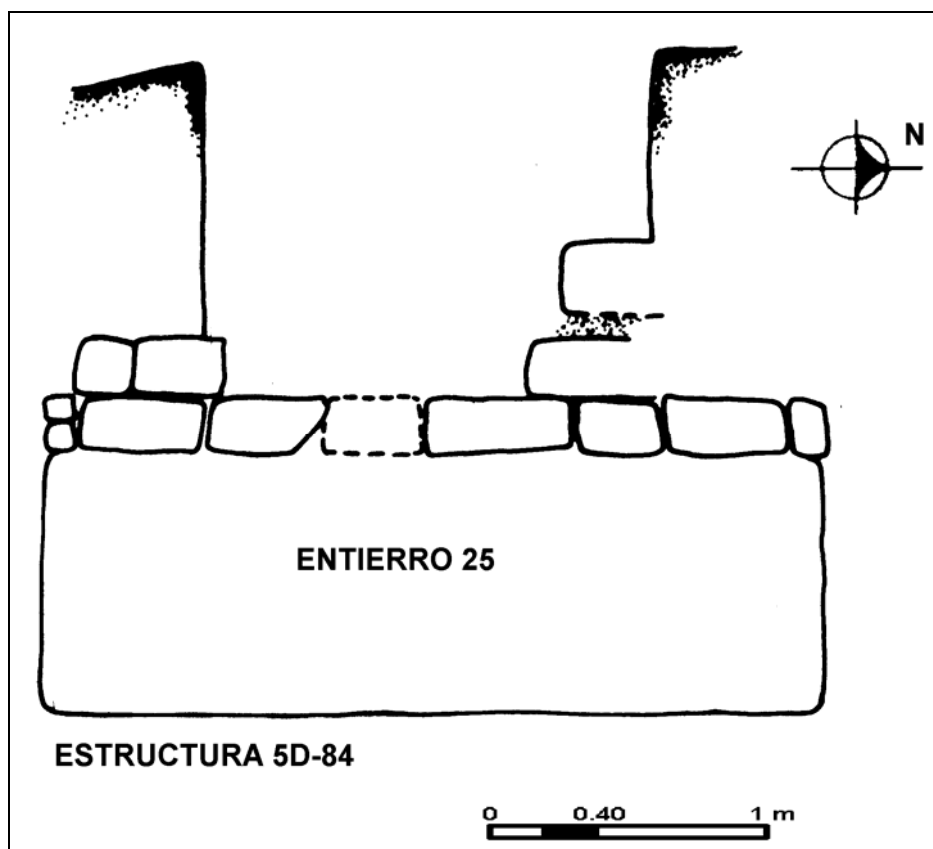
Figura 10 Corte de recinto del Entierro 25
