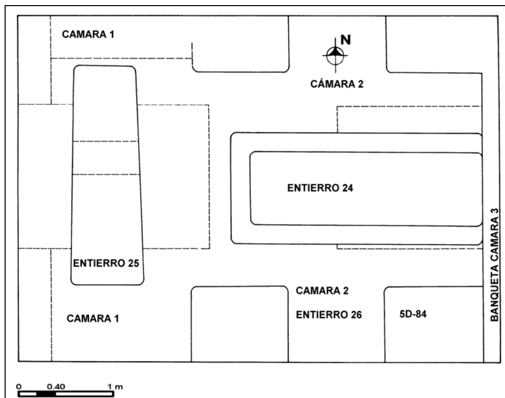
Figura 8 Planta del edificio superior mostrando posición de tres entierros, 5D-84
