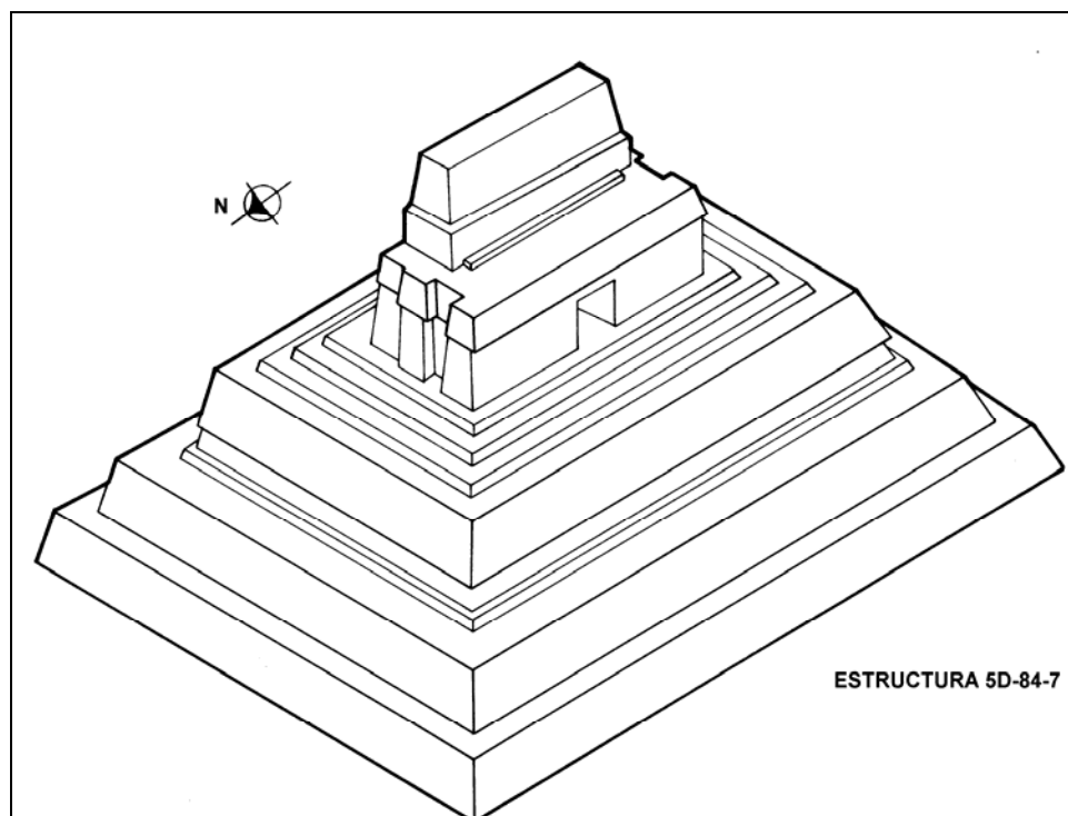
Figura 21 Modelo constructivo para la última etapa de la Estructura 5D-84
