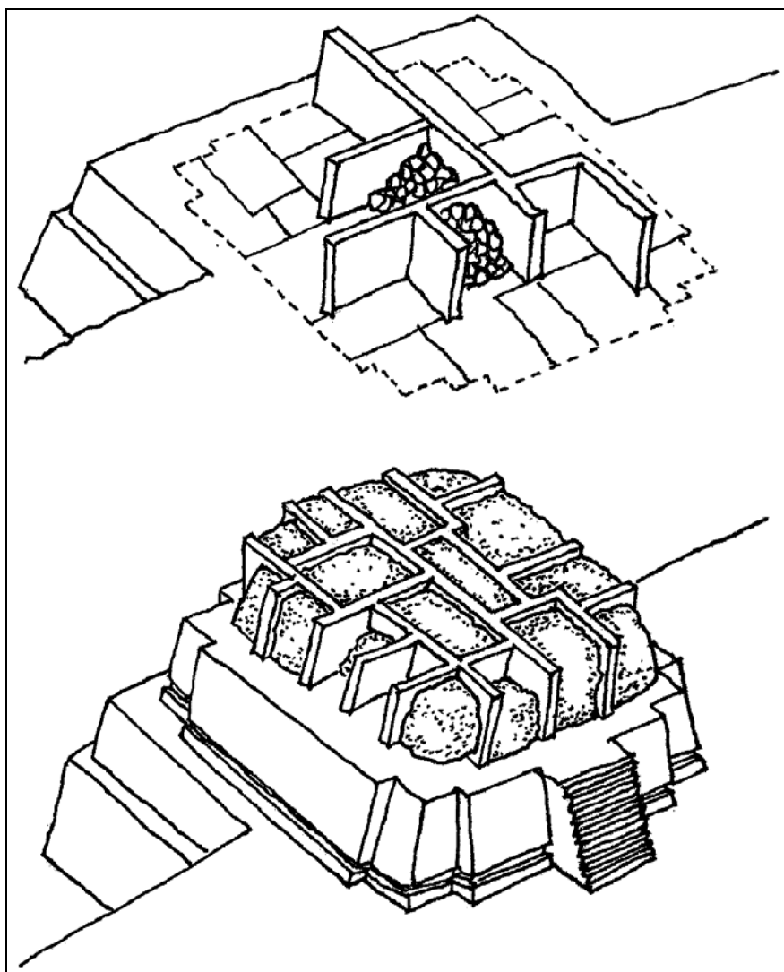
Figura 1 Esquema del sistema constructivo de cajuelas (dibujo G. Muñoz)
