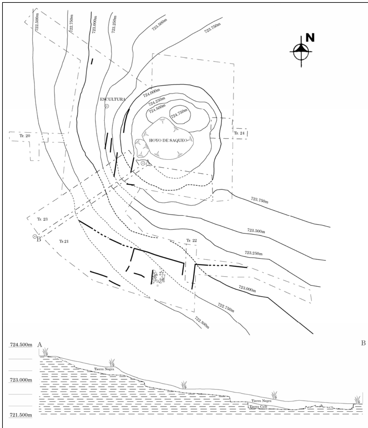
Figura 3 Planta y perfil de la Estructura 3 y concentración de piedra
