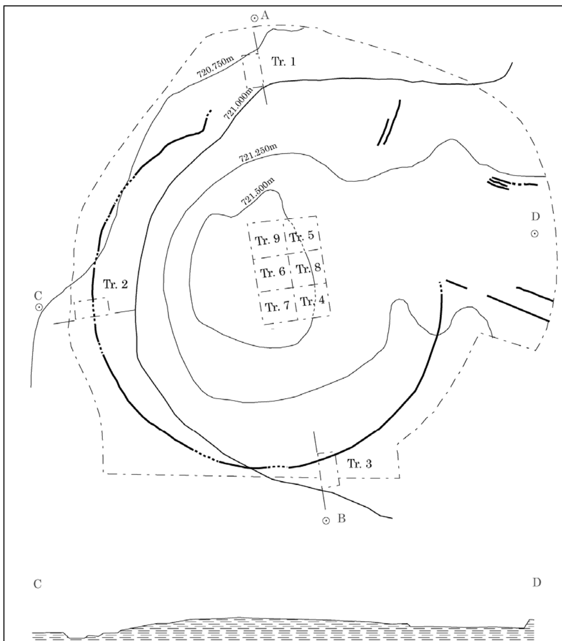
Figura 2 Planta y perfil de la Estructura 1
