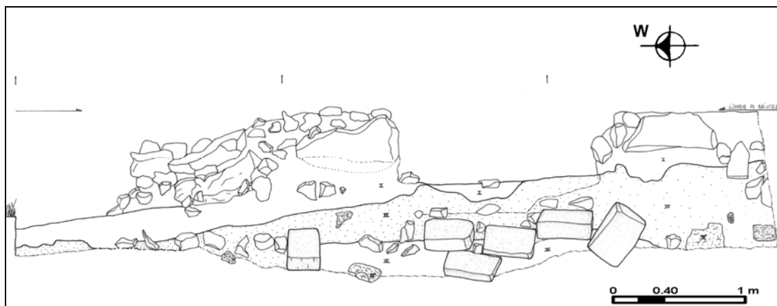
Figura 4 Vista de corte de la Subestructura del Cabildo: I. Tierra café con pómez; II. Tierra Blanca; III. Tierra blanca mezclada con tierra café (relleno); IV. Barro quemado.
