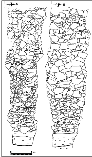
Figura 8 Perfil oeste y norte, PN64E-1, cumbre de K-5-3
