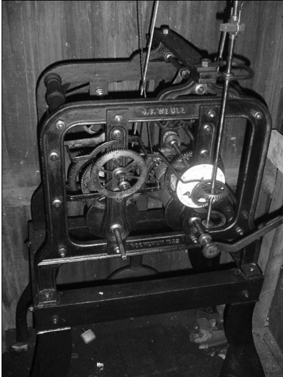
Figura 10 Reloj construido en el año de 1895 por la Casa Bockhenen, siendo su fabricante J.L. Weul
