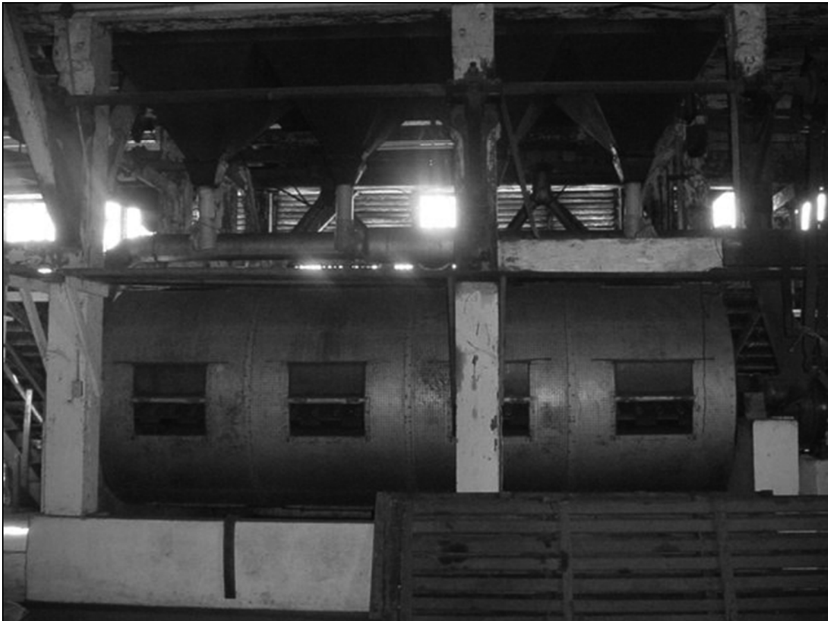
Figura 3 Secadora de café Guardiola
