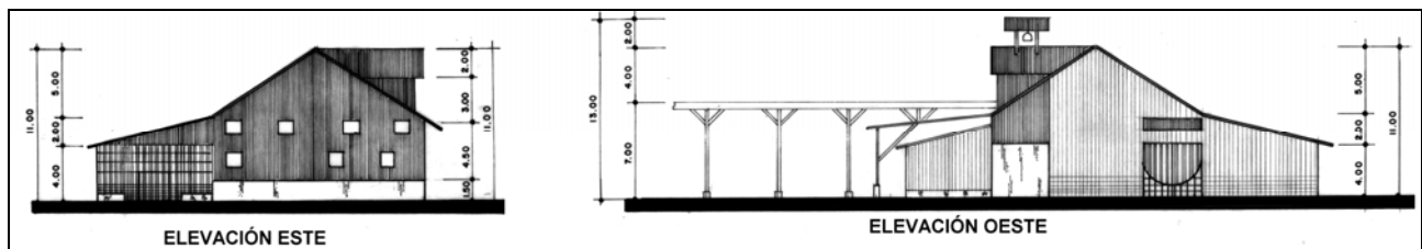
Figura 7 Elevaciones Este y Oeste del Taller de Máquinas
