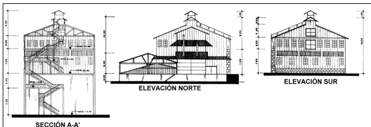
Figura 4 Elevaciones del Beneficio de Café: a) Sección A-A'; b) Elevación Norte; c) Elevación Sur
