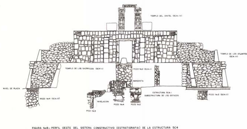
Figura 2 Corte de la Estructura 5C4
