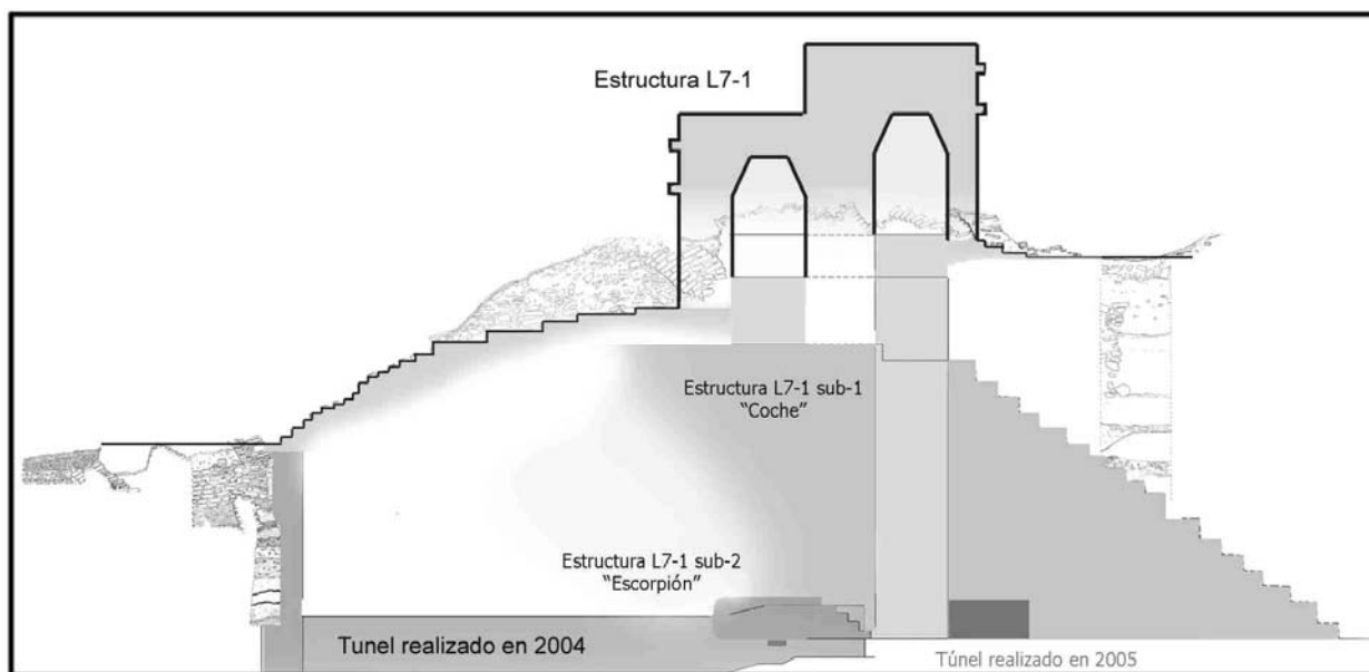
Figura 3 Esquema de las subestructuras de la Acrópolis de Cancun
