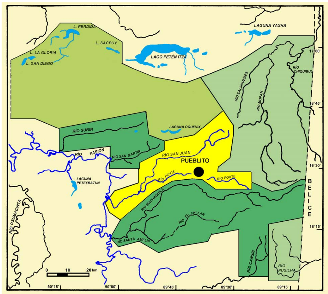
Figura 2 Cuenca del río Poxte
